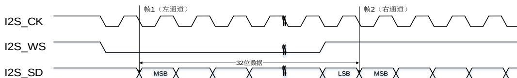
图 21-14. I2S 飞利浦标准时序图（DTLEN=10, CHLEN=1, CKPL=1）
