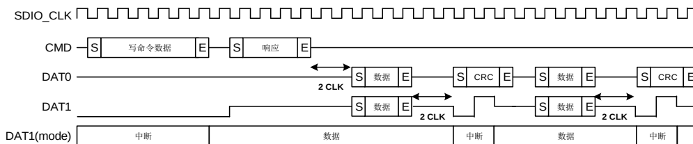
图 24-18. 4 位模式下多块写中断周期时序
