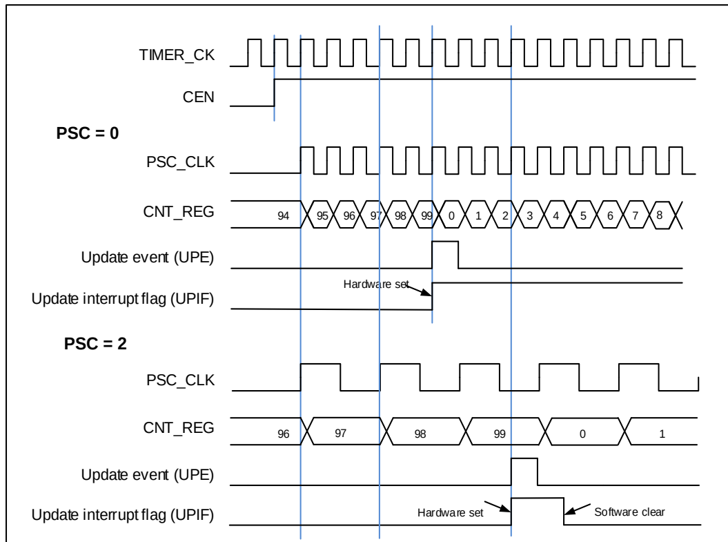
图 18-34. 向上计数时序图, PSC=0/2
