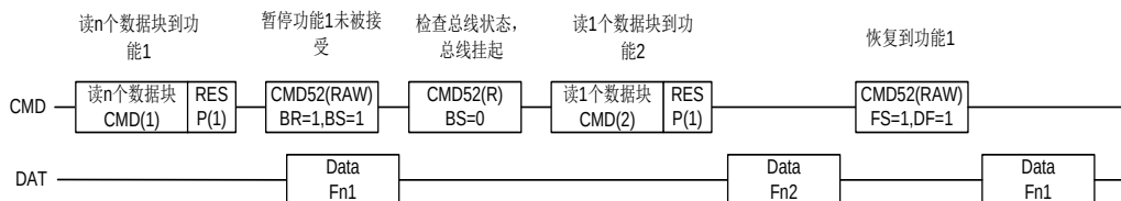
图 24-14. 在功能 1 的多块读周期期间插入功能 2 读周期
