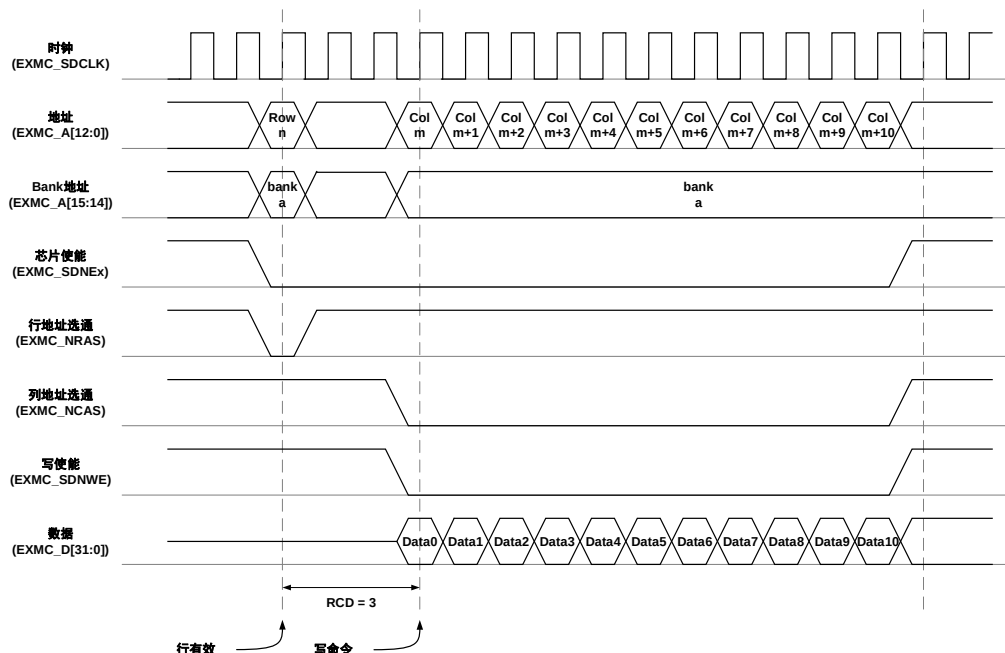
图 25-32. 突发写操作
