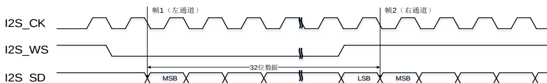
图 21-13. I2S 飞利浦标准时序图（DTLEN=10, CHLEN=1, CKPL=0）
