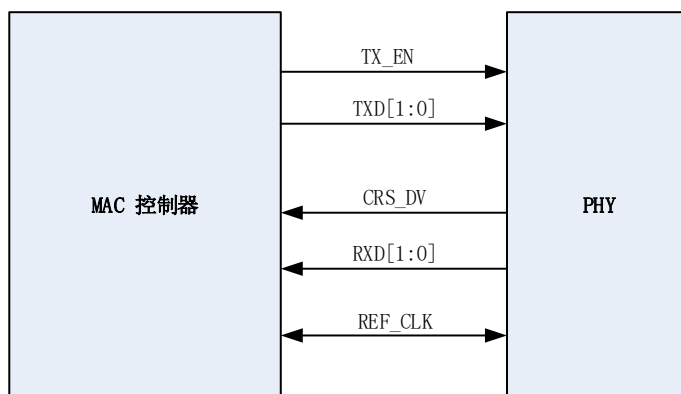
图 27-5. 精简媒体独立接口(RMII)信号线
