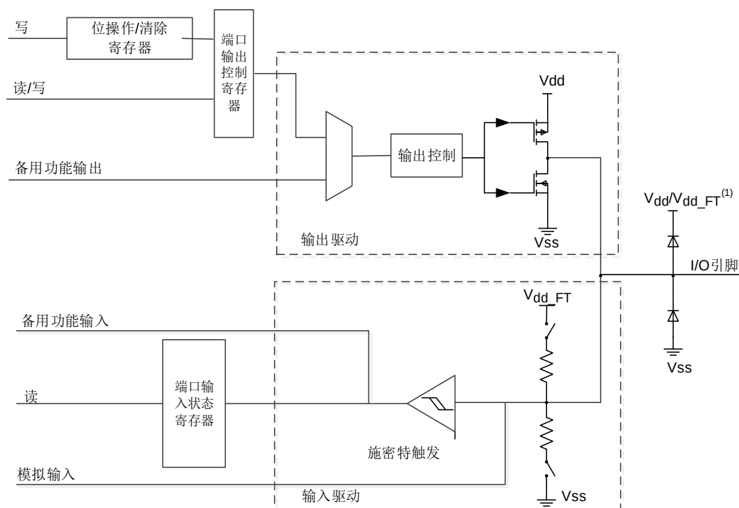
图 7-1. 标准 I/O 端口和 5V 兼容 I/O 口的基本结构
