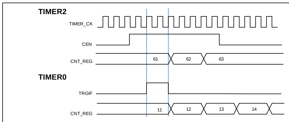
图 18-29. 用定时器2的使能信号启动定时器0
