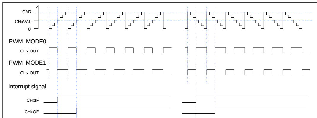
图 18-16. EAPWM 时序图
