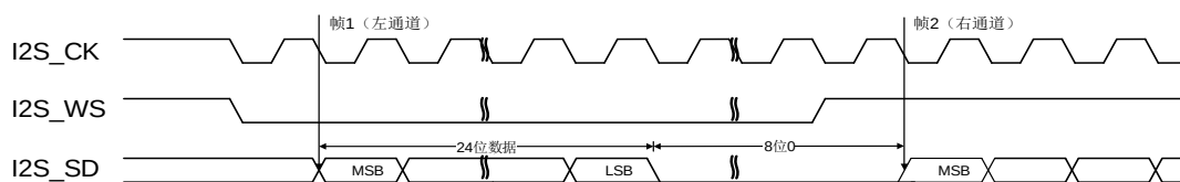
图 21-16. I2S 飞利浦标准时序图 (DTLEN=01, CHLEN=1, CKPL=1)
