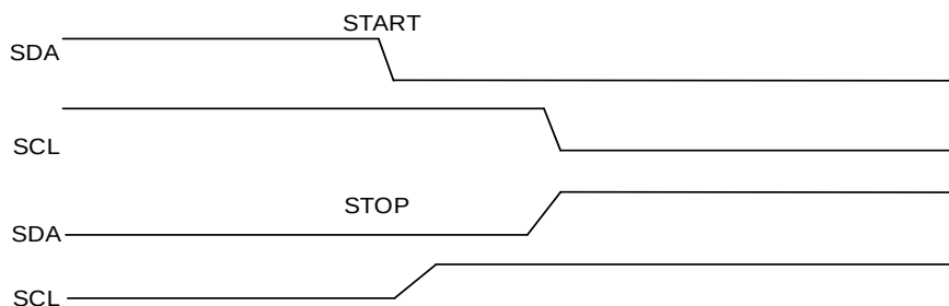
图 20-3. 开始和停止信号
