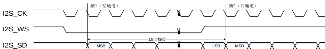
图 21-12. I2S 飞利浦标准时序图（DTLEN=00, CHLEN=0, CKPL=1）
