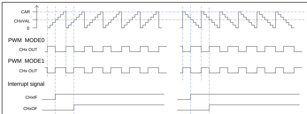
图 18-60. CAPWM 时序图
