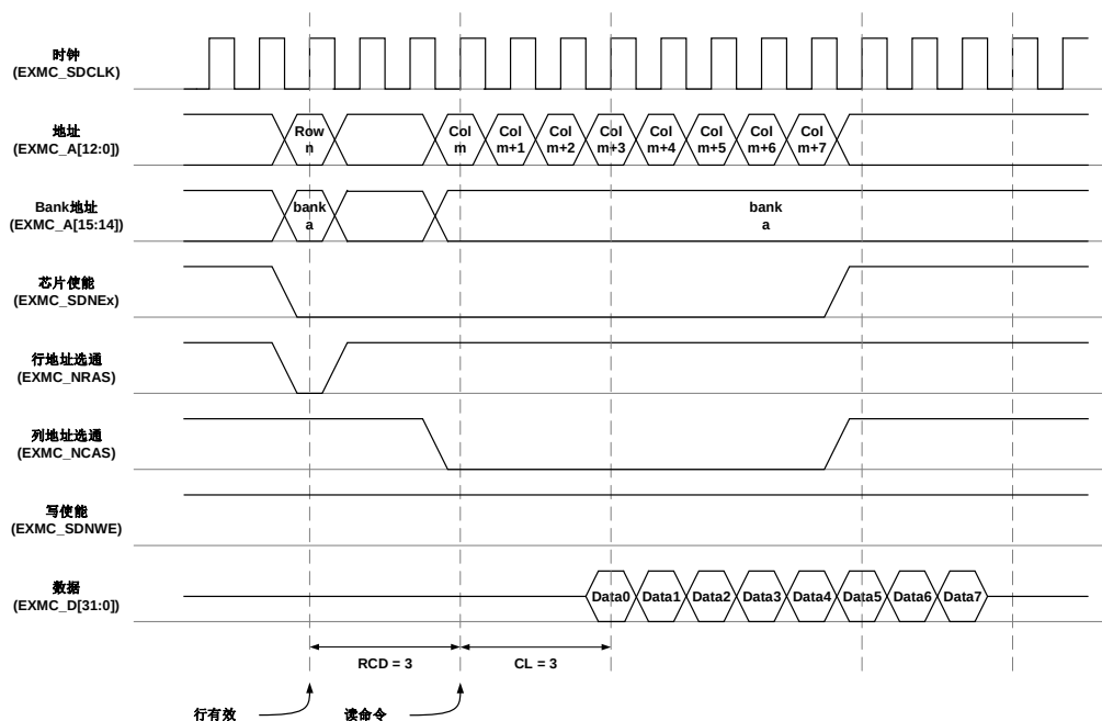
图 25-30. 突发读操作
