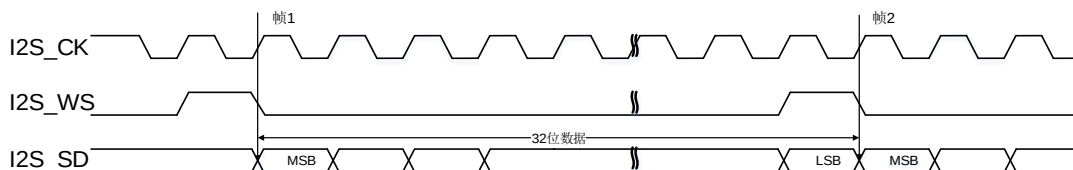
图 21-34. PCM 标准短帧同步模式时序图 (DTLEN=10, CHLEN=1, CKPL=1)
