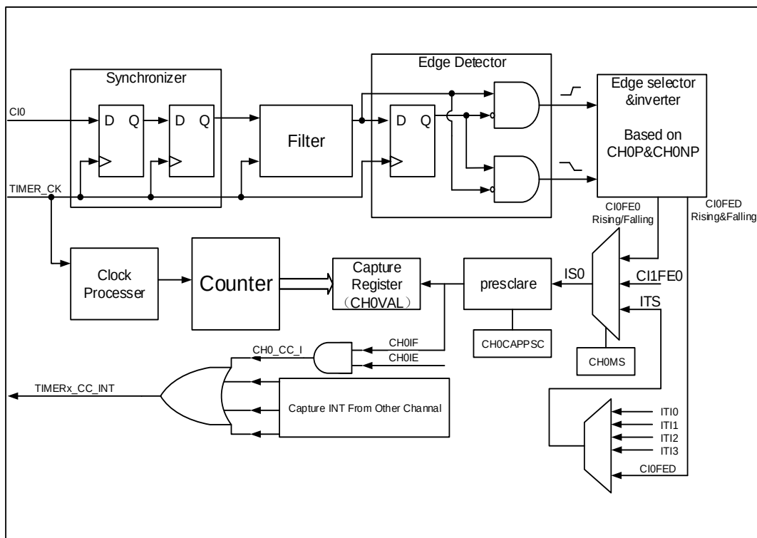
图 18-39. 通道输入捕获原理
