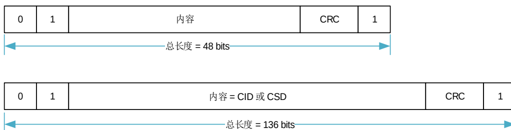
图 24-8. 响应令牌格式
