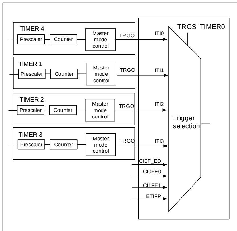
图 18-28. 定时器 0 主/从模式的例子
