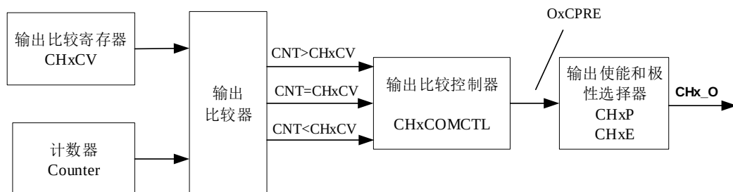
图 18-57. 通道输出比较原理 (x=0,1)
