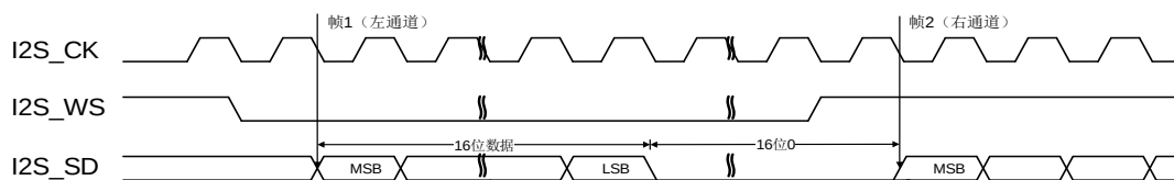
图 21-17. I2S 飞利浦标准时序图 (DTLEN=00, CHLEN=1, CKPL=0)
