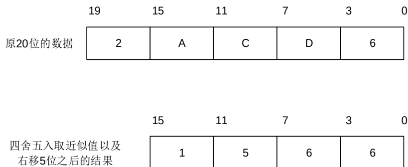
图 14-12. 右移 5 位和取整的数例
