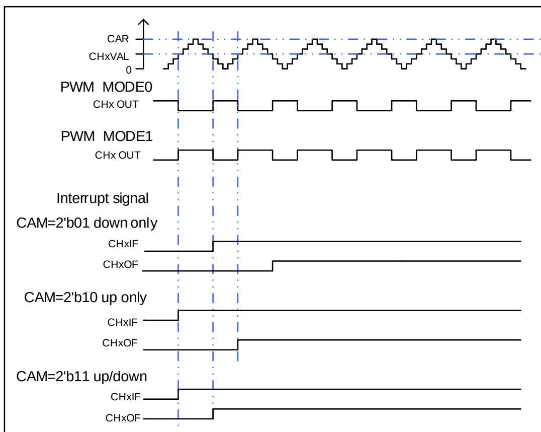
图 18-43. CAPWM 时序图
