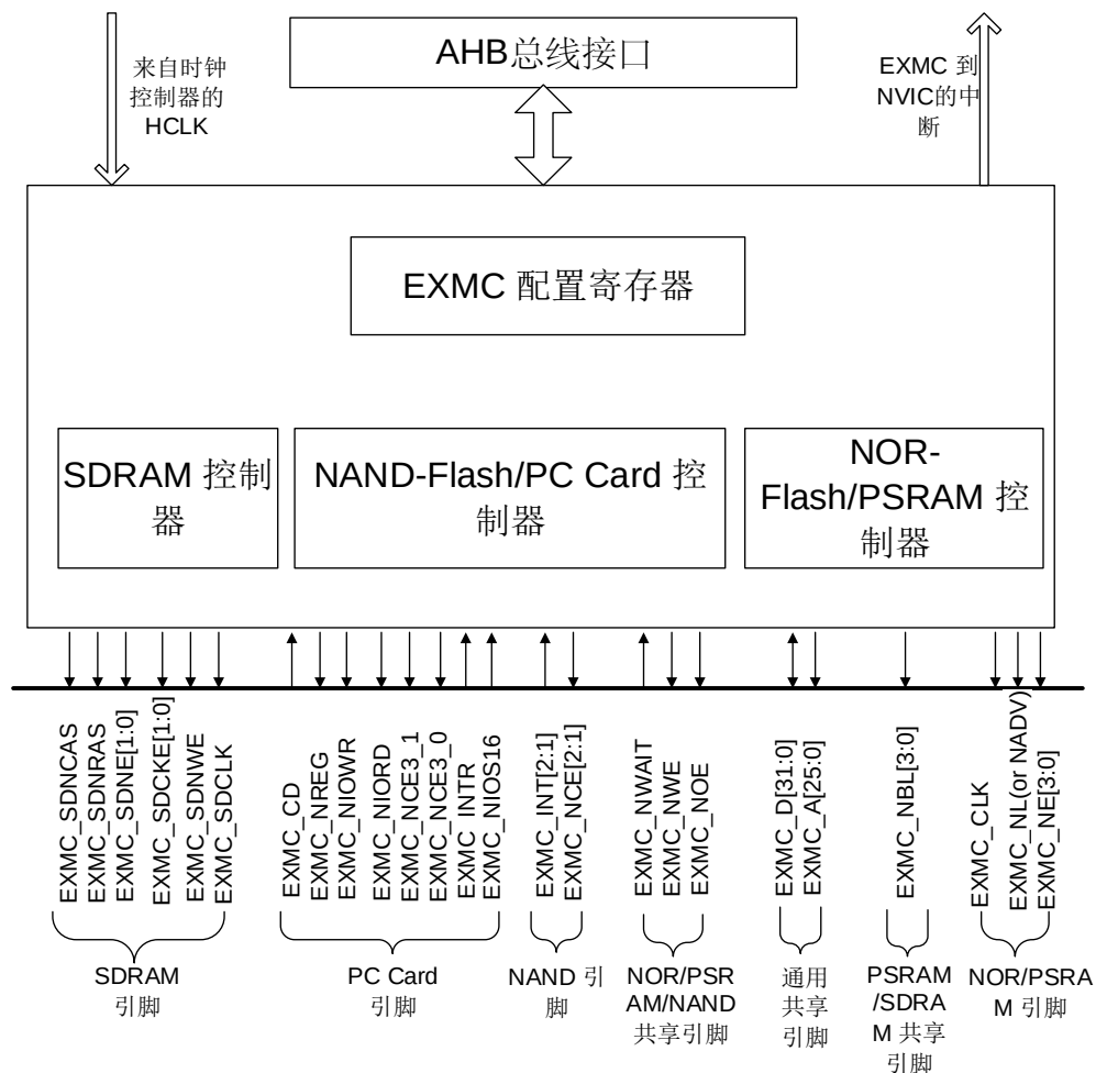
图 25-1. 系统架构
