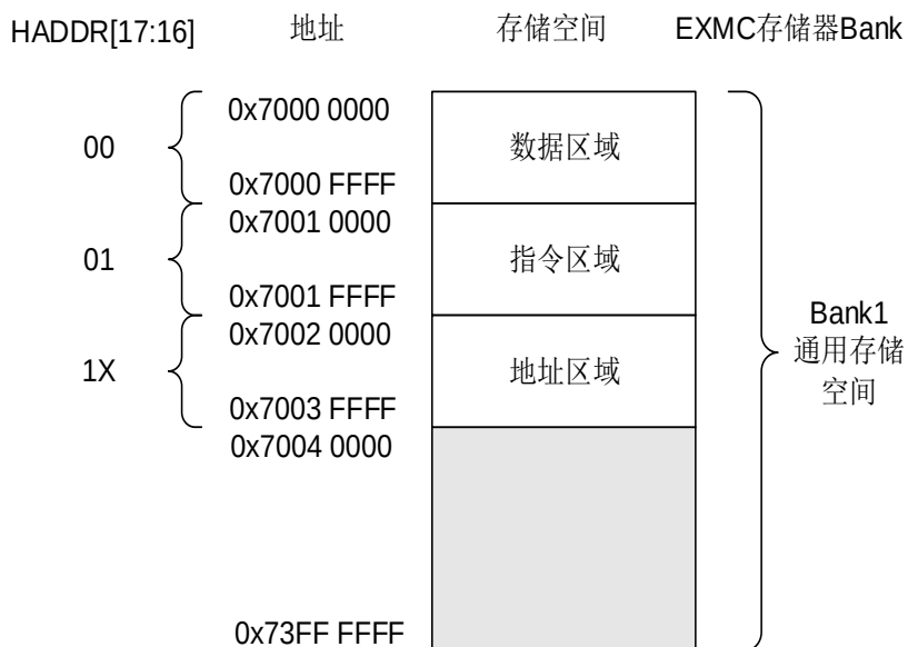
图 25-5. Bank1 通用空间
