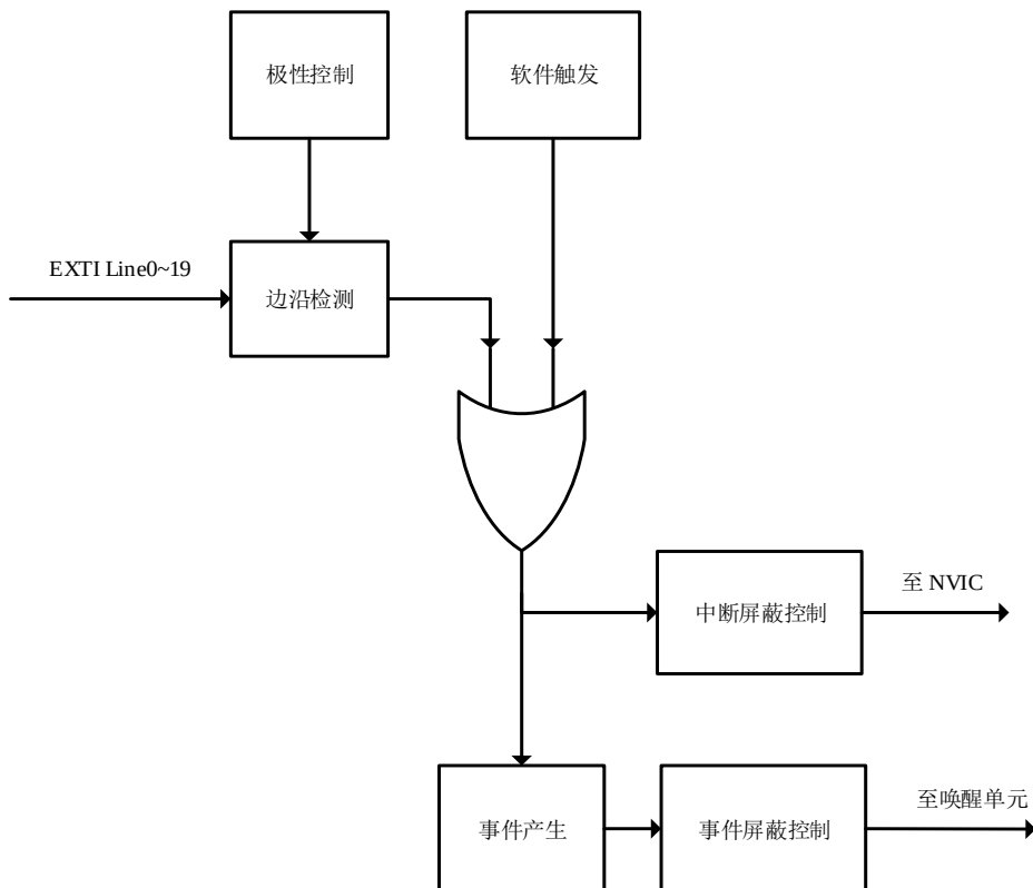
图 6-1. EXTI 框图
