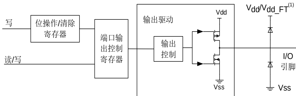
图 7-3. 输出配置
