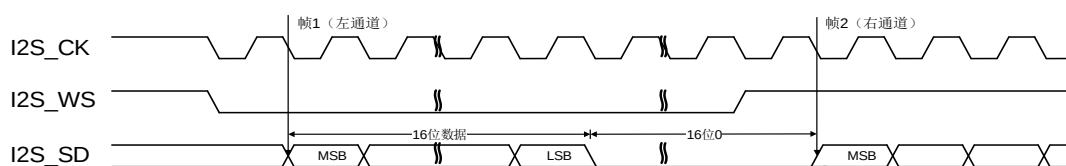
图 21-18. I2S 飞利浦标准时序图 (DTLEN=00, CHLEN=1, CKPL=1)
