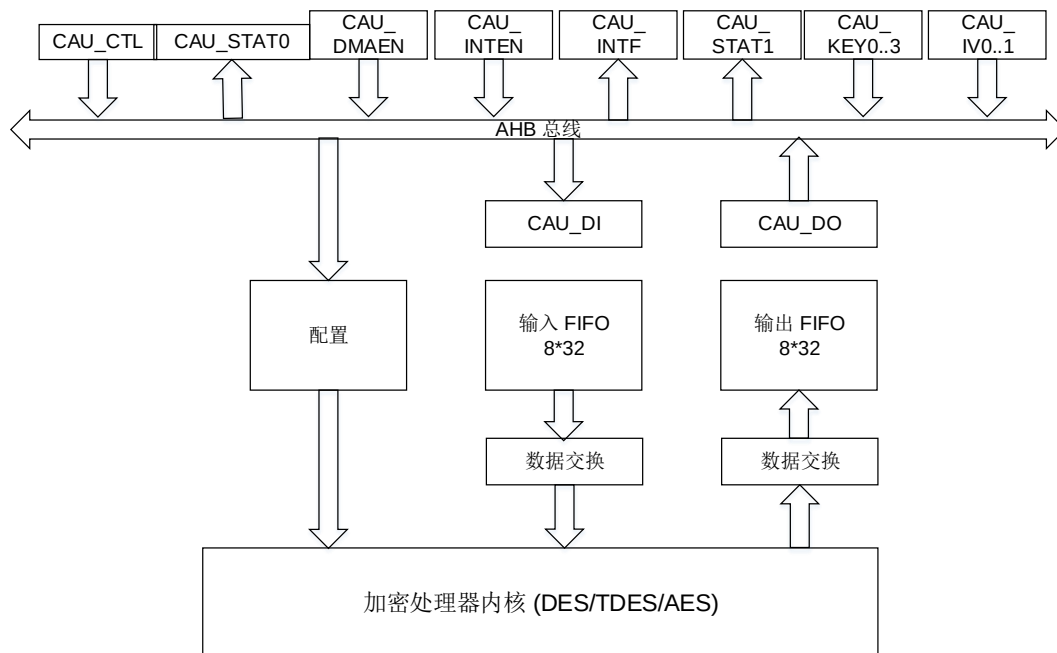
图 10-3. CAU 框图
