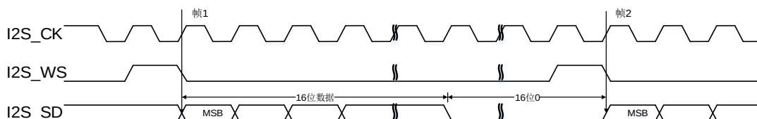
图 21-38. PCM 标准短帧同步模式时序图 (DTLEN=00, CHLEN=1, CKPL=1)
