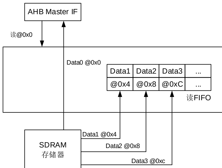
图 25-33. FIFO 未命中时的读访问（BRSTRD=1，CL=2，SDCLK=2，PIPED=2）
