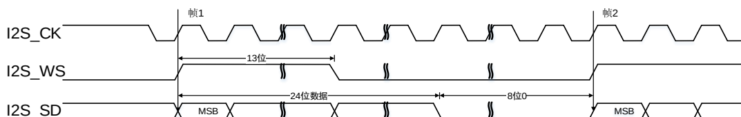
图 21-44. PCM 标准长帧同步模式时序图 (DTLEN=01, CHLEN=1, CKPL=1)
