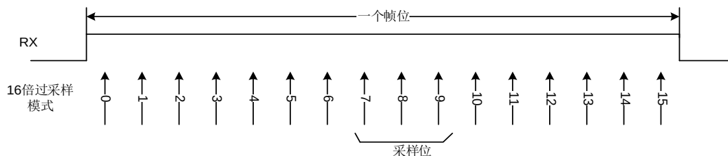
图 19-4. 过采样方式接收一个数据位
