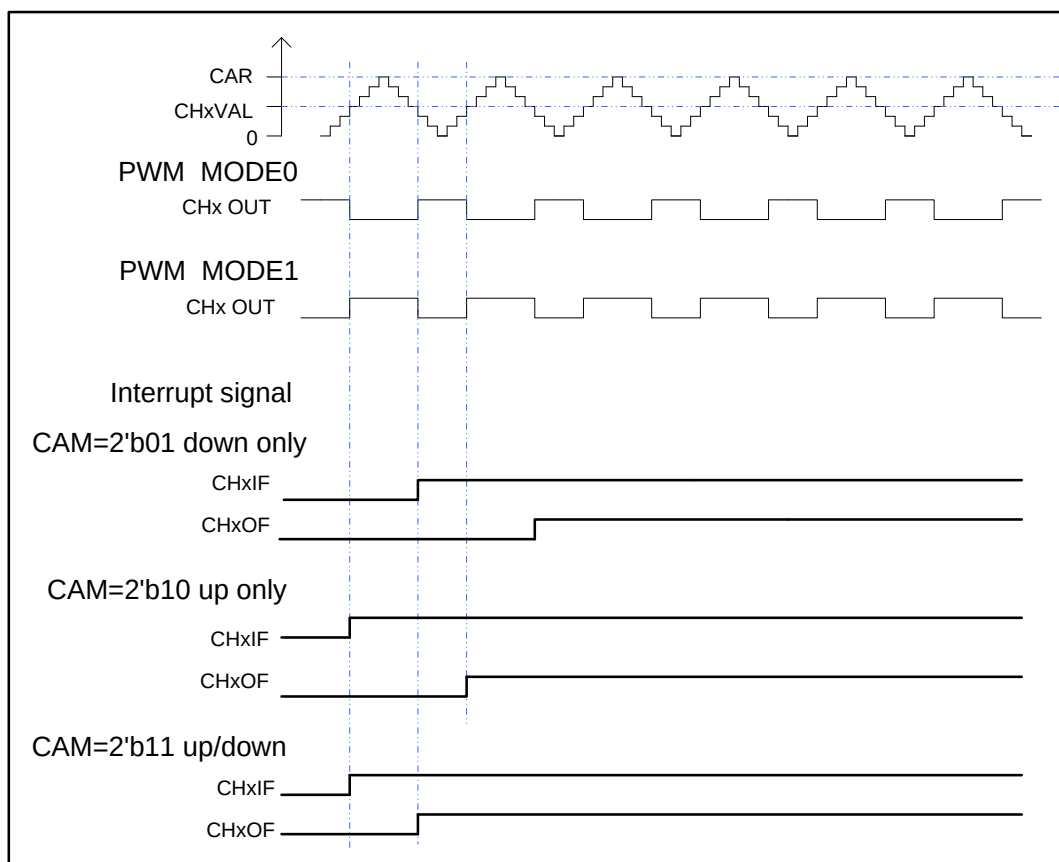
图 18-60. CAPWM 时序图
