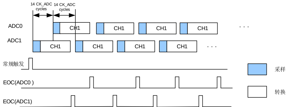
图 14-16. 常规序列通道上的慢速交叉模式
