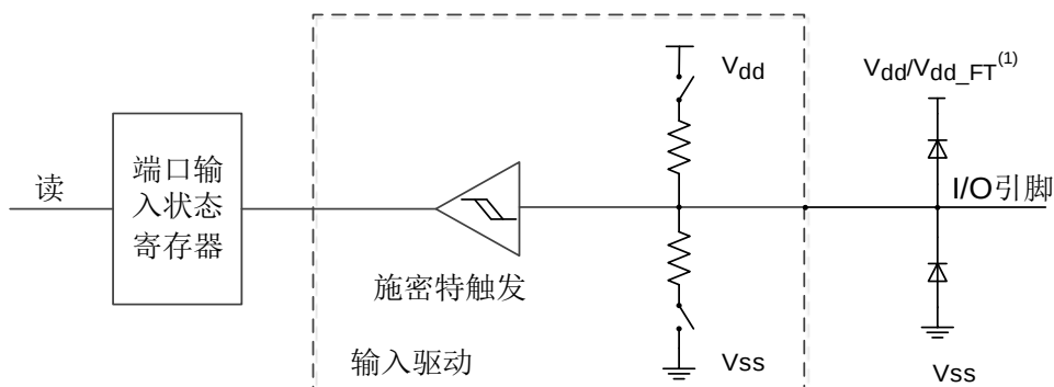
图 7-2. 输入配置
