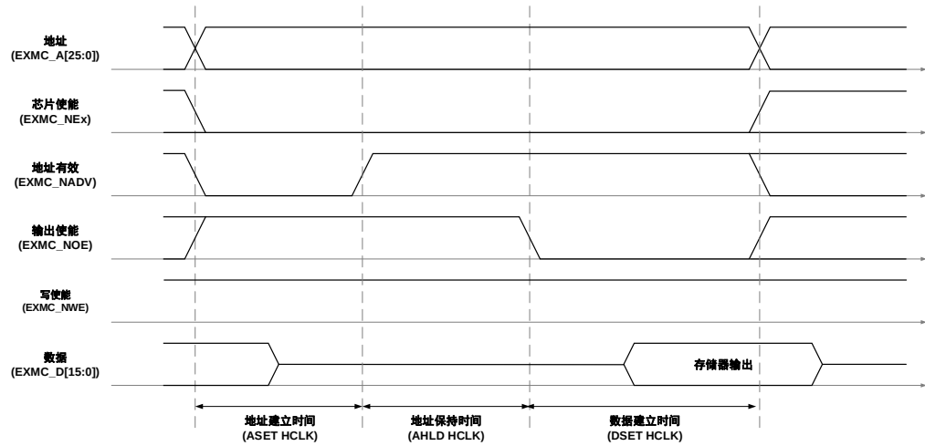
图 25-17. 模式 D 写时序
