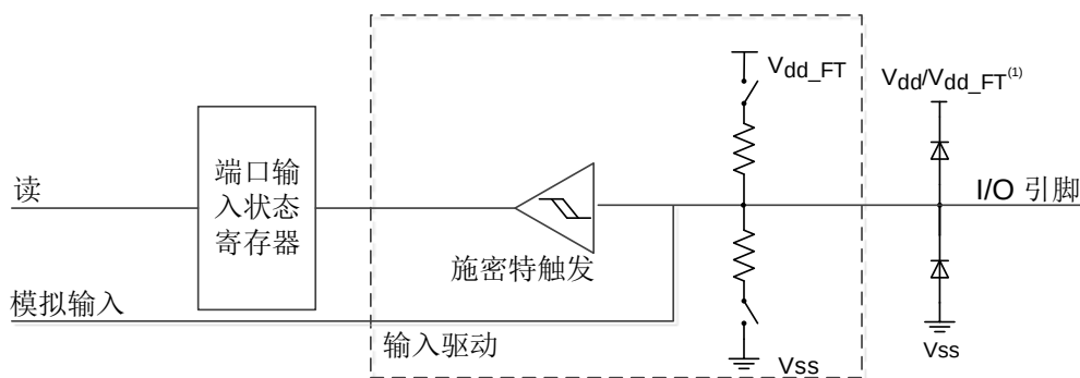
图 7-4. 模拟配置
