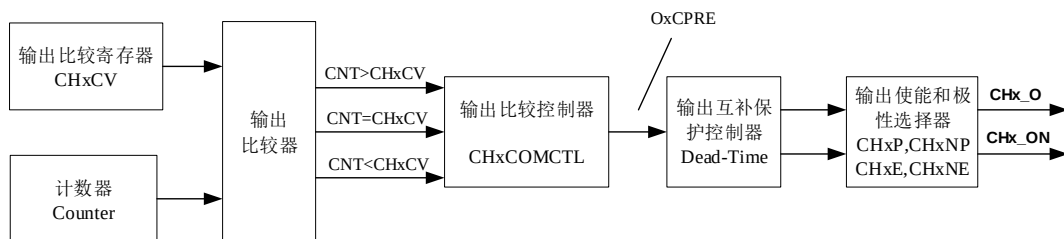
图 18-14. 通道输出比较原理
