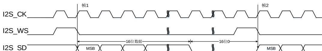
图 21-37. PCM 标准短帧同步模式时序图 (DTLEN=00, CHLEN=1, CKPL=0)
