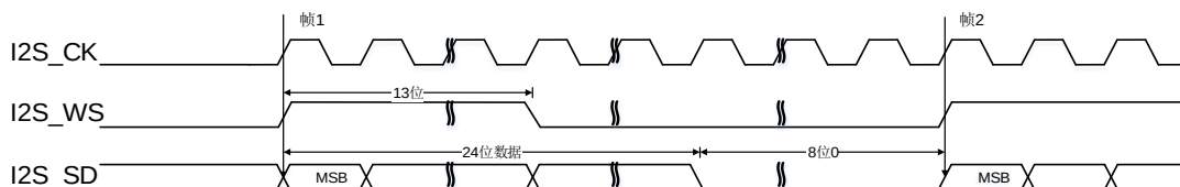
图 21-43. PCM 标准长帧同步模式时序图 (DTLEN=01, CHLEN=1, CKPL=0)
