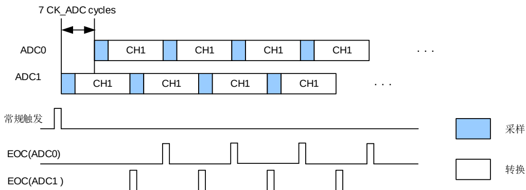
图 14-15. 常规序列上的快速交叉模式（两个 ADC 的 CTN=1）
