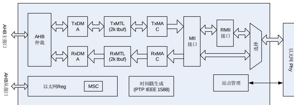
图 27-1. 以太网模块框图
