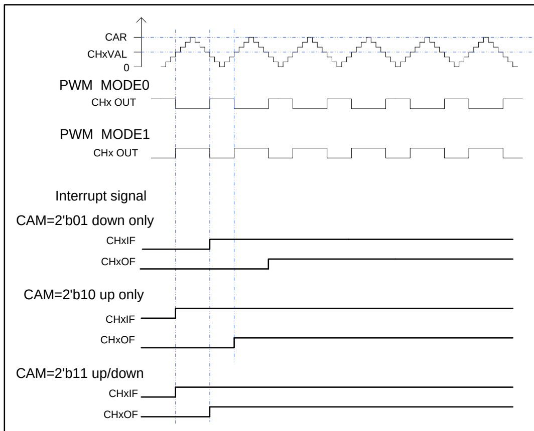
图 18-17. CAPWM 时序图
