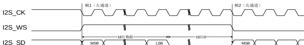
图 21-26. MSB 对齐标准时序图 (DTLEN=00, CHLEN=1, CKPL=1)
