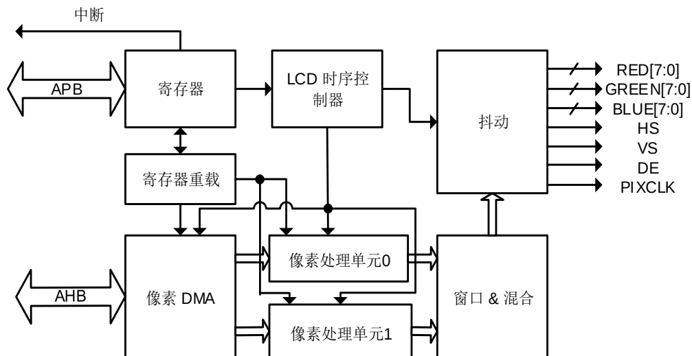
图 23-1. TLI 模块框图
