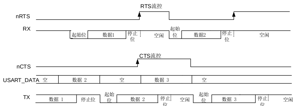
图 19-8. 硬件流控制
