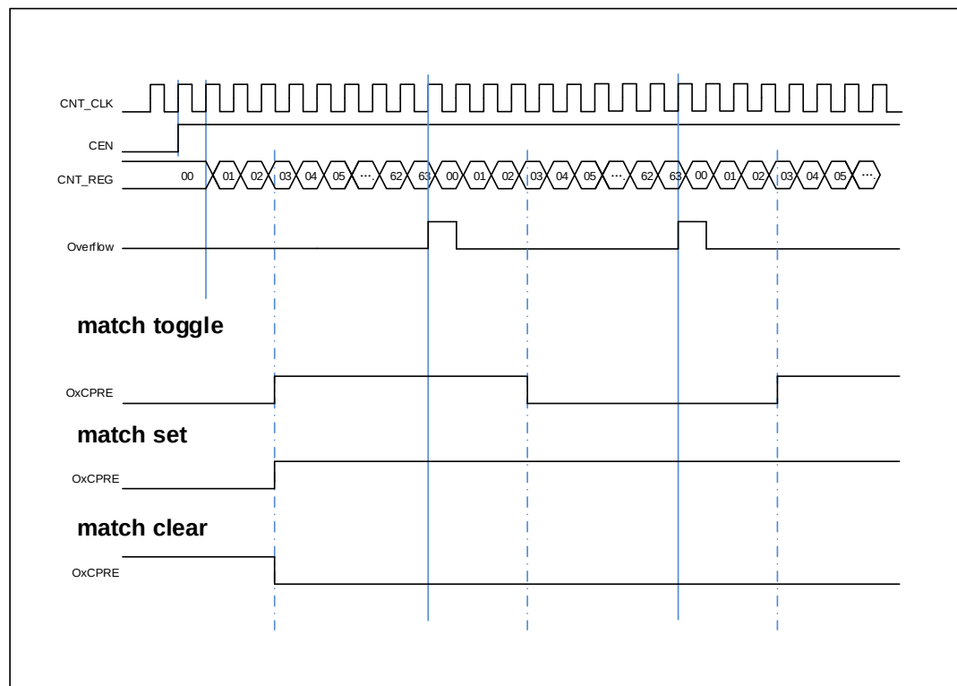
图 18-74. 三种输出比较模式
