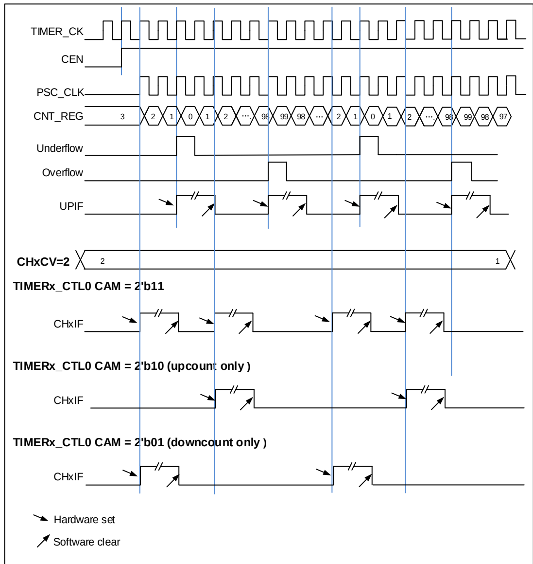
图 18-8. 中央对齐计数模式计数器时序图
