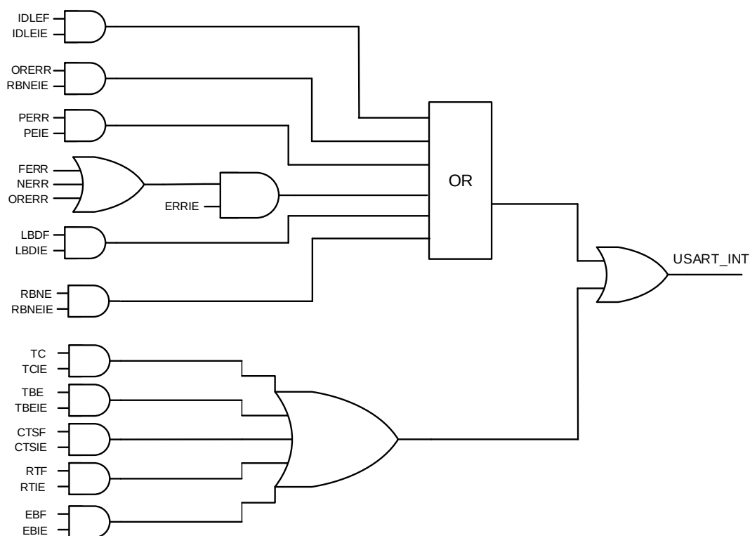
图 19-16. USART 中断映射框图
