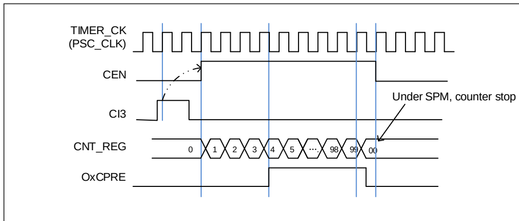
图 18-47. 单脉冲模式，TIMERx_CHxCV = 4 TIMERx_CAR=99
