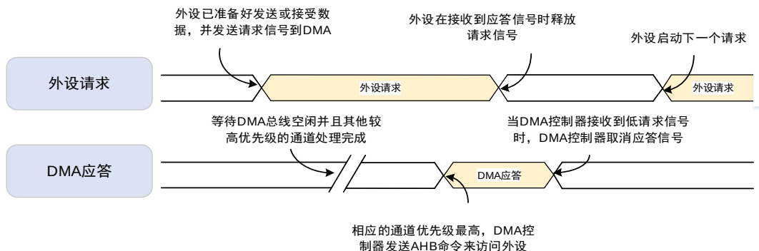
图 11-5. 握手机制
