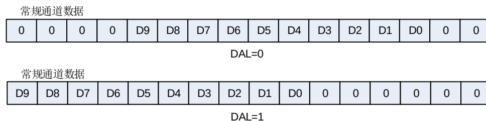
图 14-8. 10 位数据存储模式
