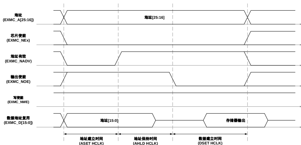
图 25-18. 复用模式读时序
