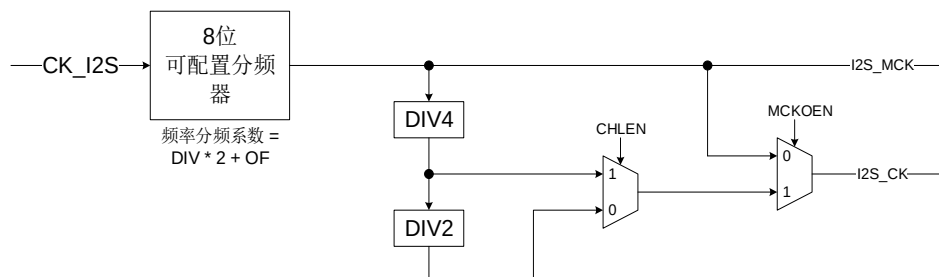
图 21-47. I2S 时钟生成结构框图
