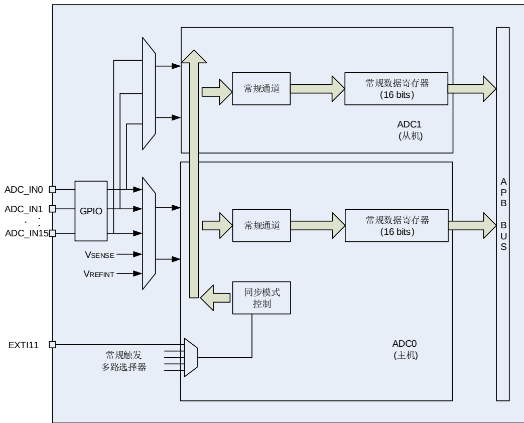
图 14-13. ADC 同步框图
