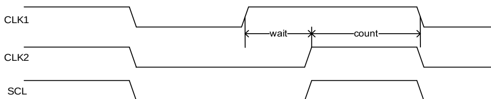
图 20-4. 时钟同步
