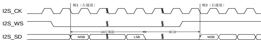
图 21-15. I2S 飞利浦标准时序图 (DTLEN=01, CHLEN=1, CKPL=0)
