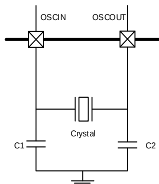
图5-3. HXTAL时钟源
