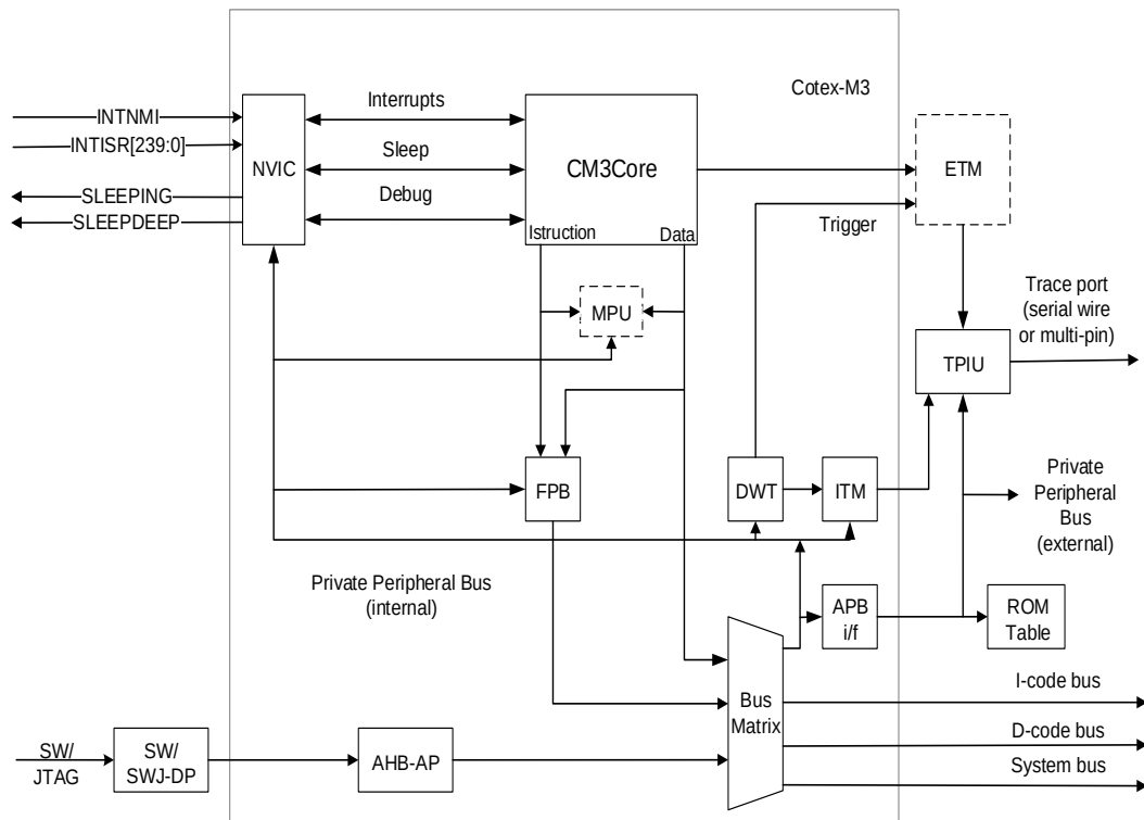
图 1-1. Cortex®-M3 结构图
