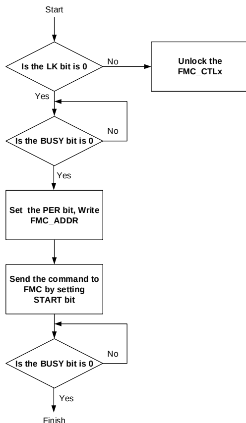
图 2-1. 页擦除操作流程
