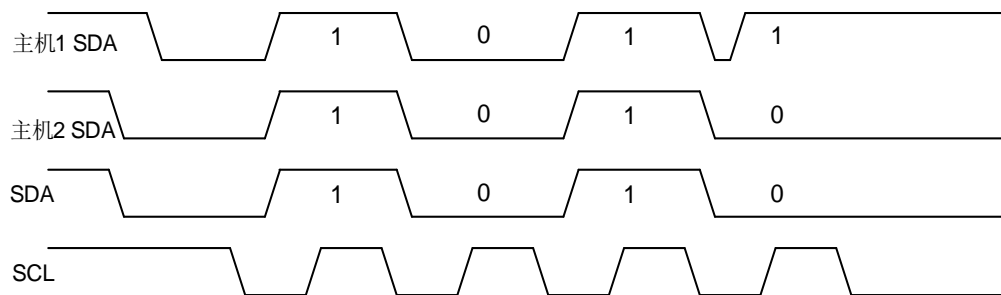
图 17-5. SDA 线仲裁
