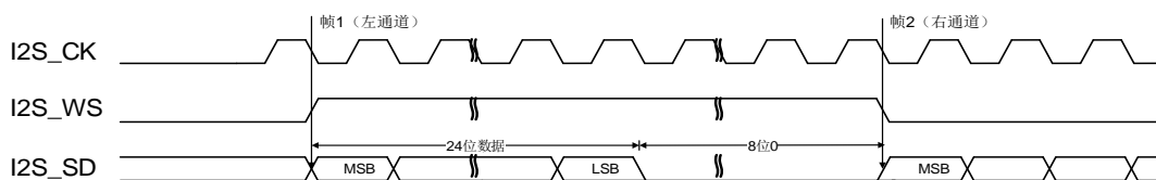
图 18-24. MSB 对齐标准时序图 (DTLEN=01, CHLEN=1, CKPL=0)
