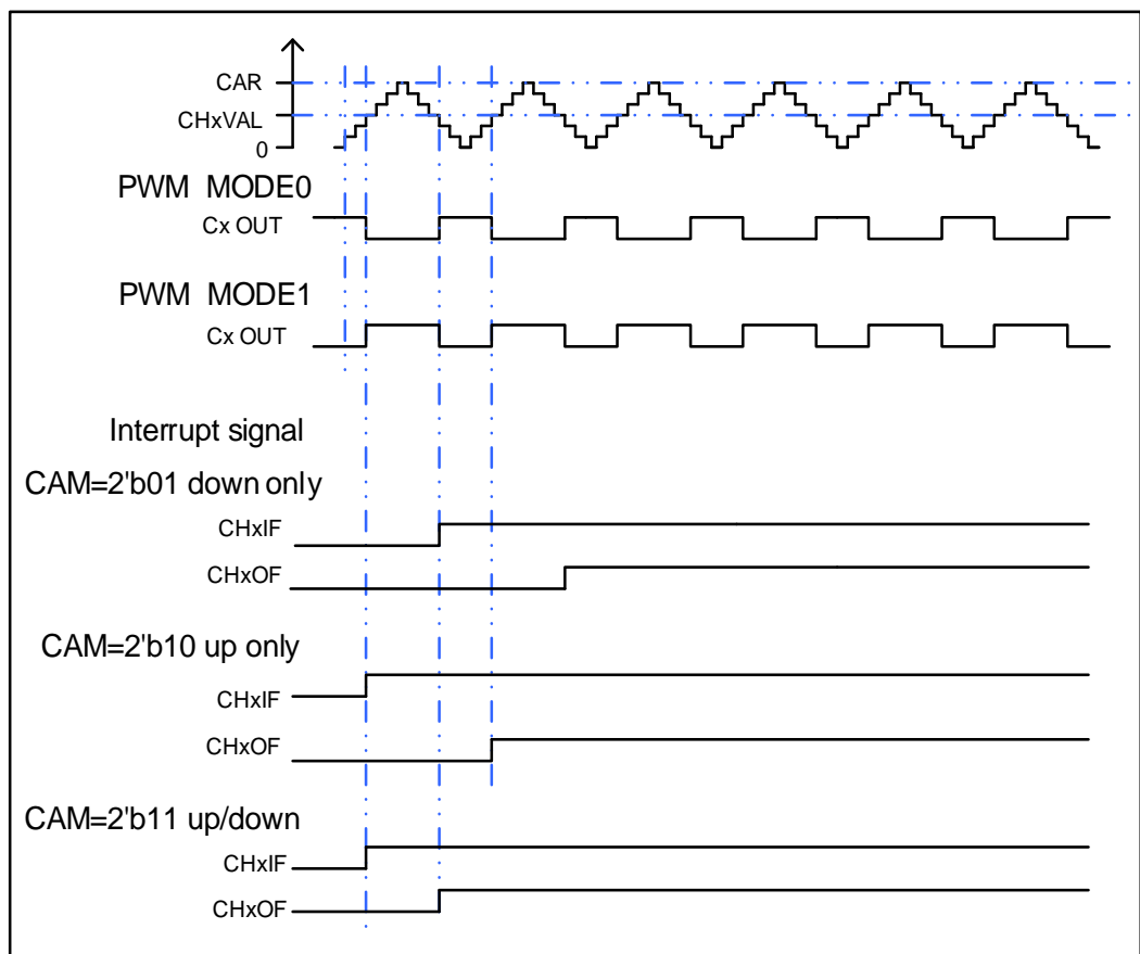
图 15-17. CAPWM 时序图
