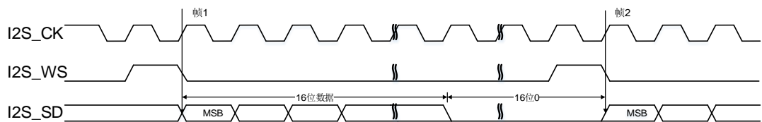
图 18-39. PCM 标准短帧同步模式时序图 (DTLEN=00, CHLEN=1, CKPL=1)
