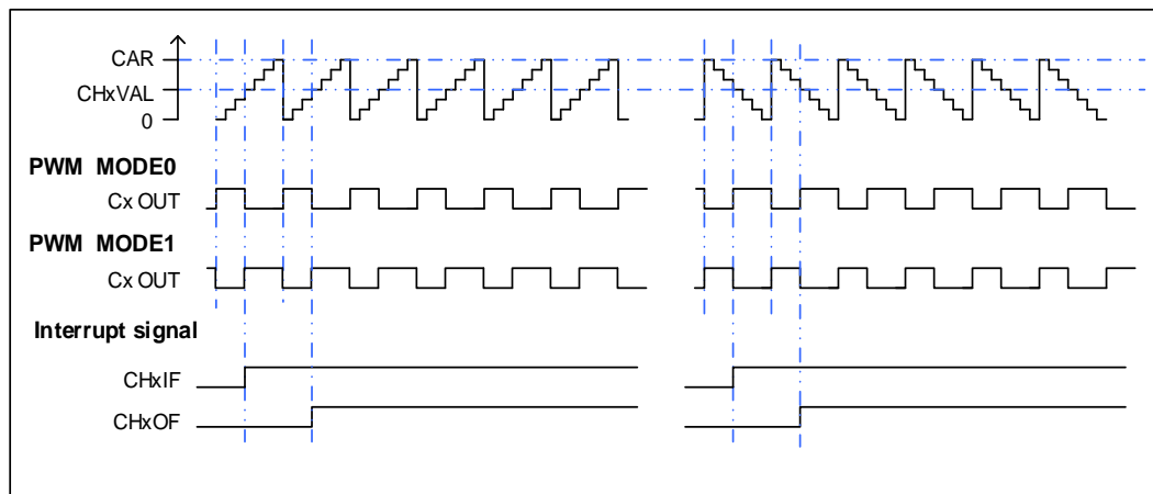
图 15-16. EAPWM 时序图
