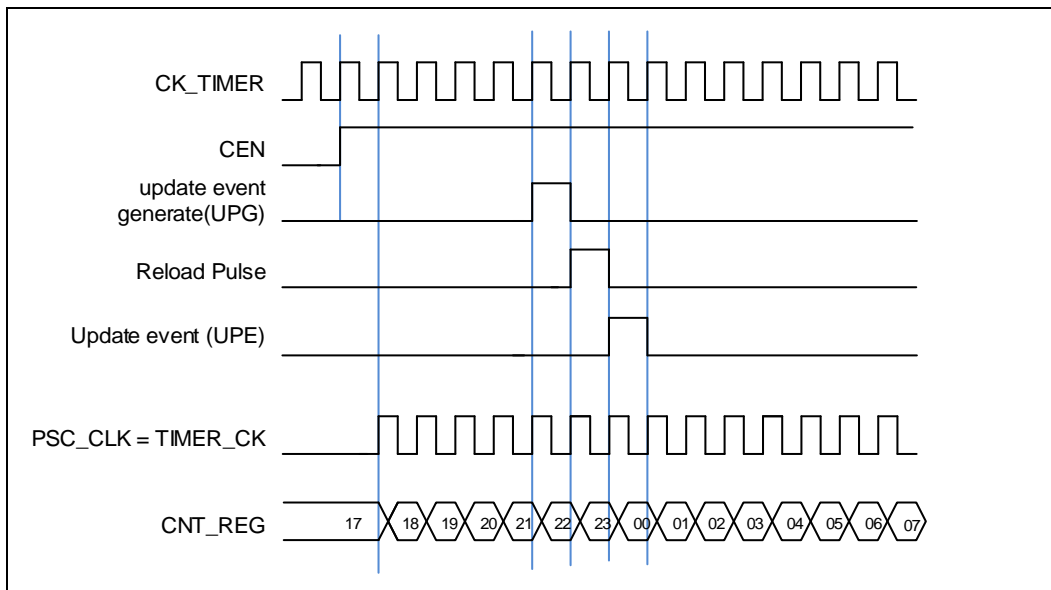
图 15-31. 内部时钟分频为 1 时，计数器的时序图
