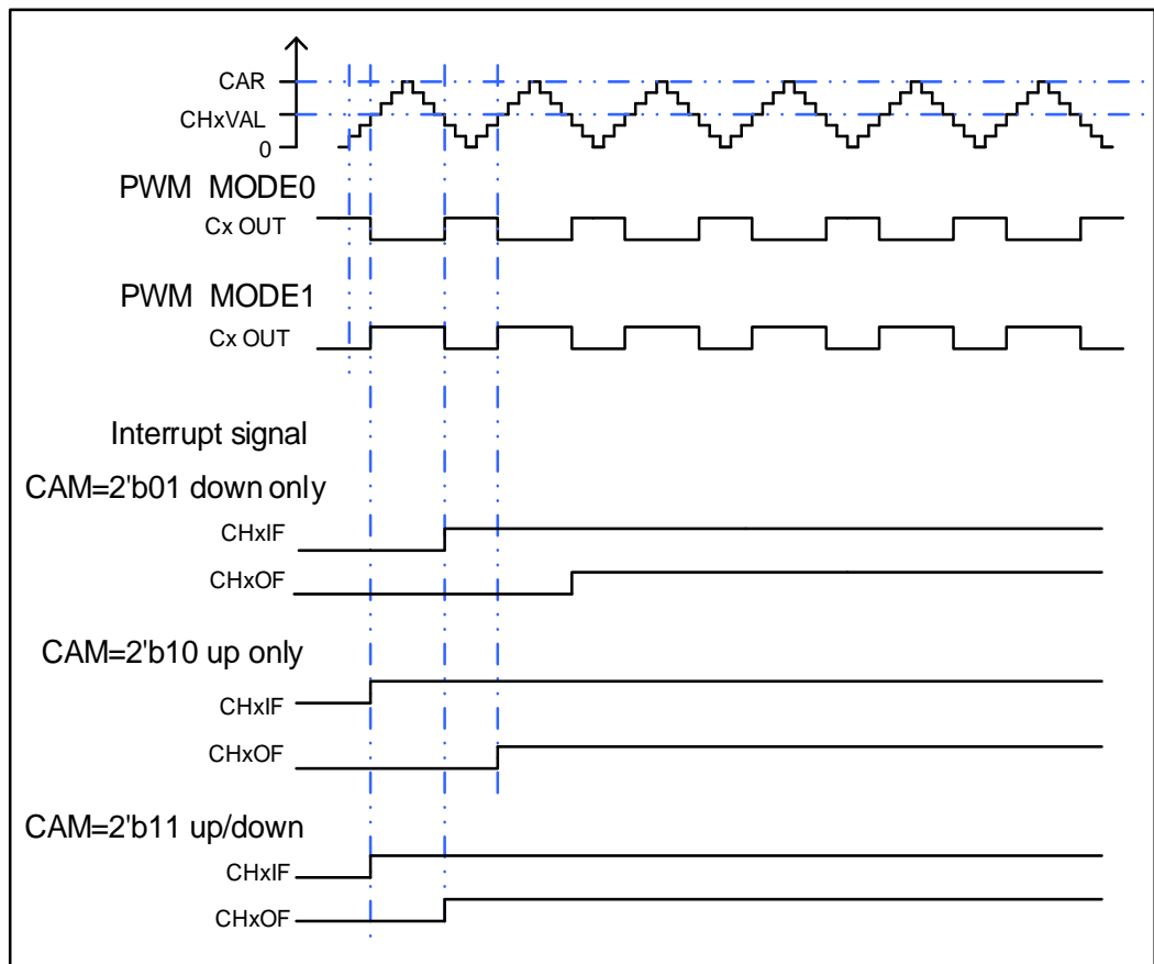
图 15-41. CAPWM 时序图
