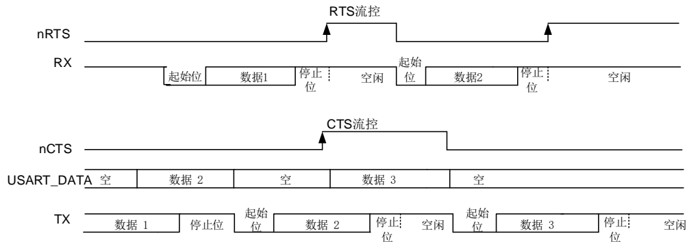
图 16-8. 硬件流控制
