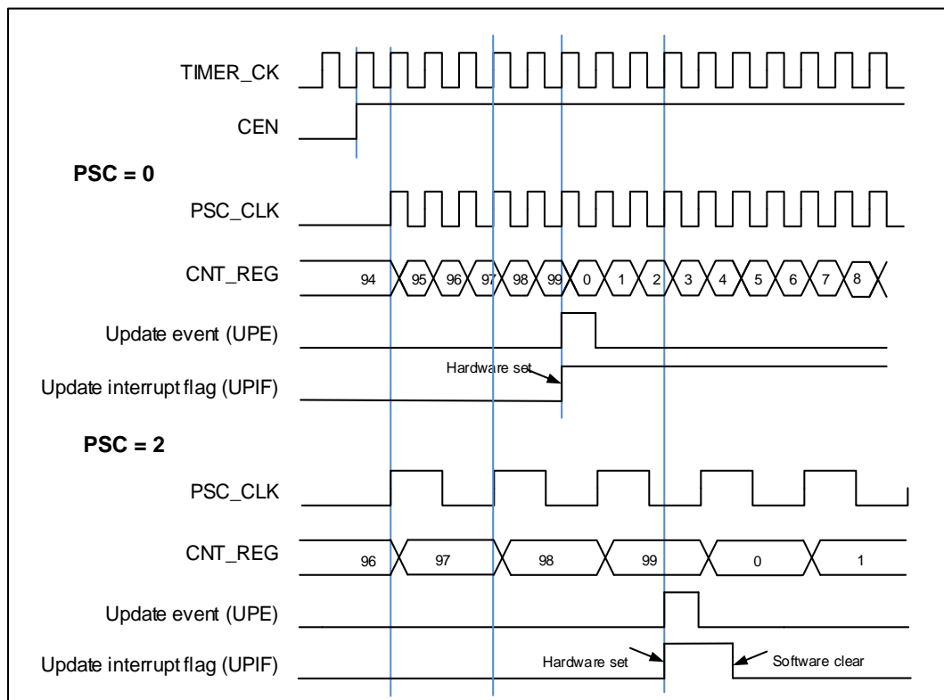
图 15-33. 向上计数时序图, PSC=0/2
