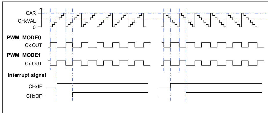
图 15-40. EAPWM 时序图
