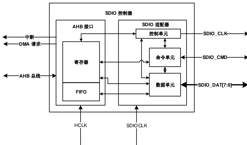
图 24-6. SDIO 框图
