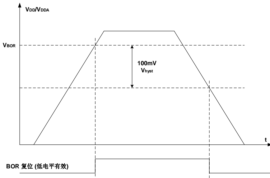
图4-2. BOR波形图
