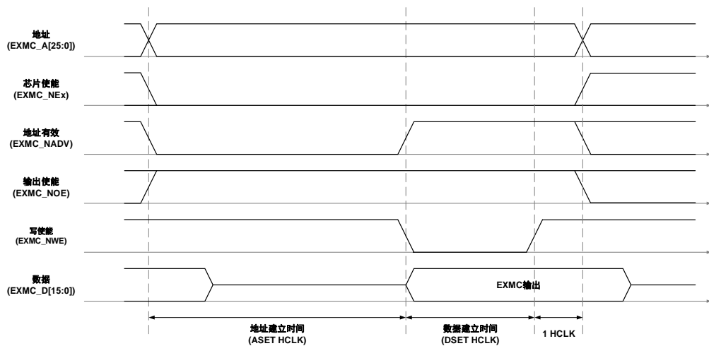
图 25-11. 模式 2 写时序
