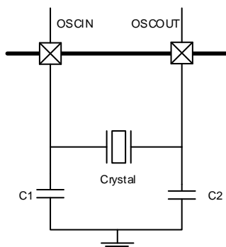
图5-3. HXTAL时钟源
