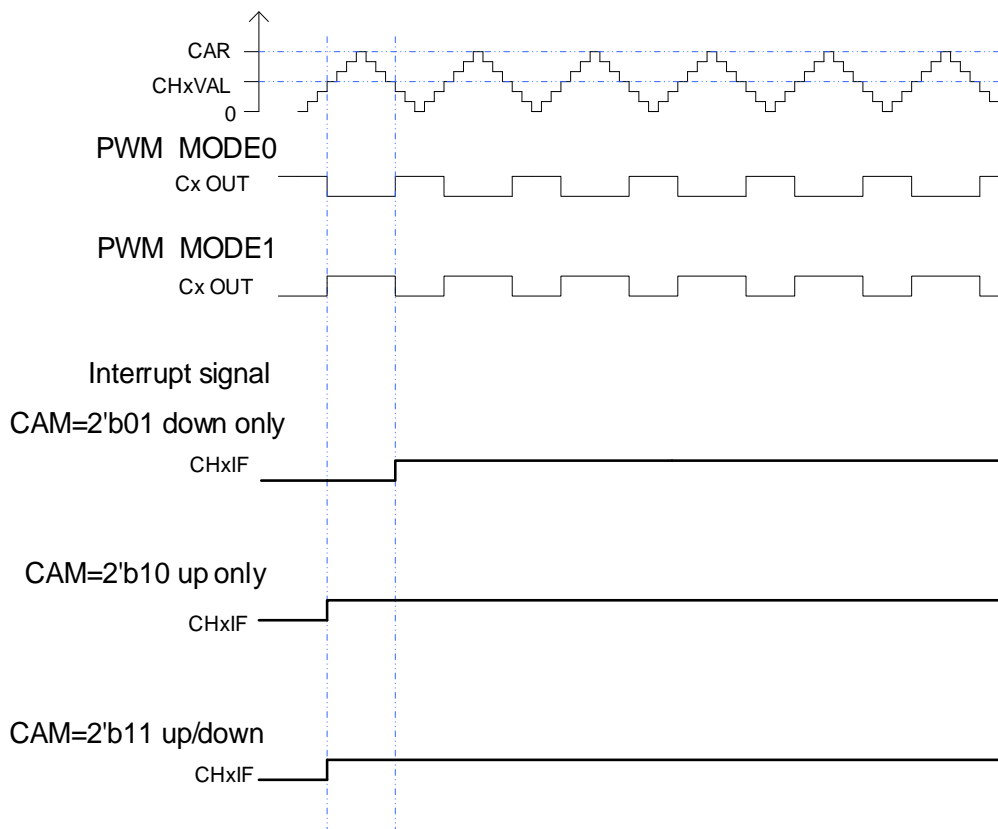
图 18-17. CAPWM 时序图
