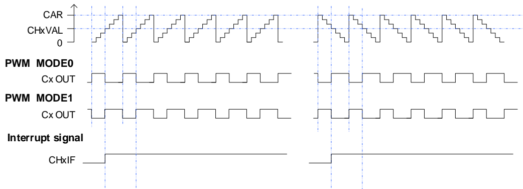
图 18-42. CAPWM 时序图
