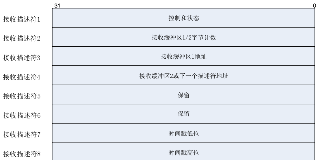
图 27-10. 增强接收描述符
