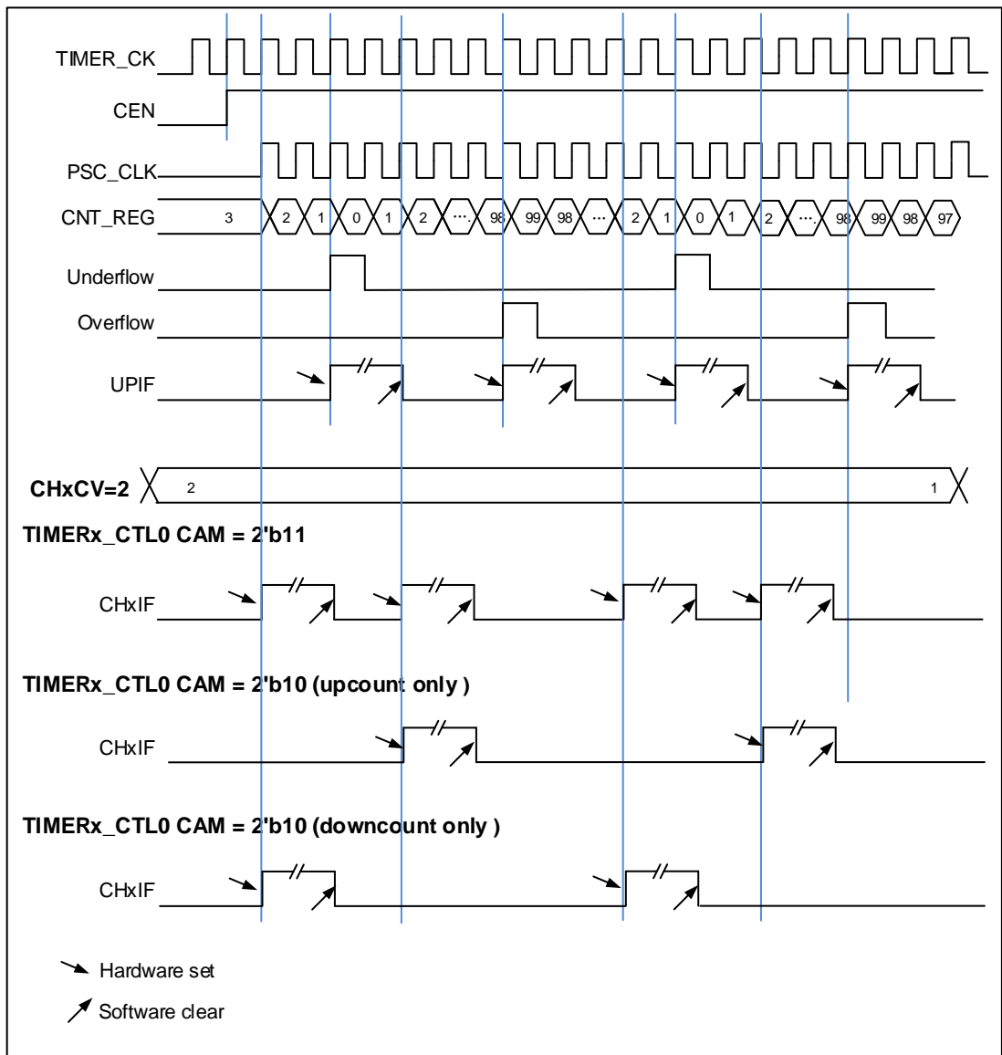
图 18-37. 中央计数模式计数器时序图
