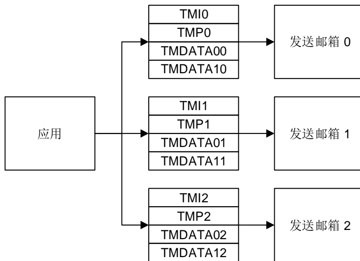
图 26-2. 发送寄存器
