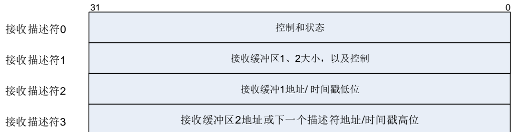
图 27-9. 常规接收描述符
