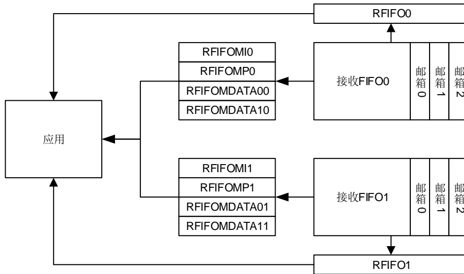
图 26-4. 接收寄存器
