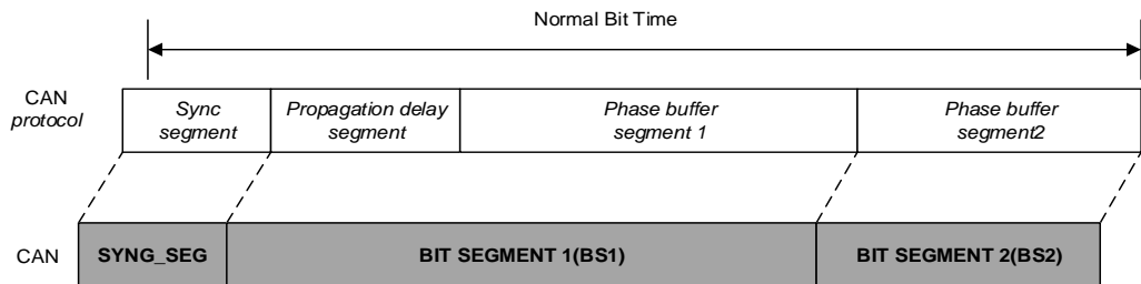
图 26-11. 位时序
