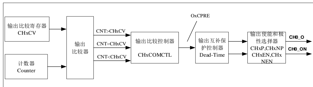
图 18-13. 输出比较原理（带有互补输出的通道， x=0,1,2 ）
