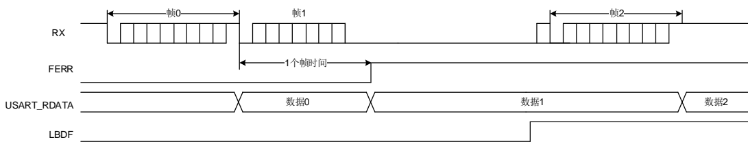
图 20-24. 数据传输过程中检测断开帧
