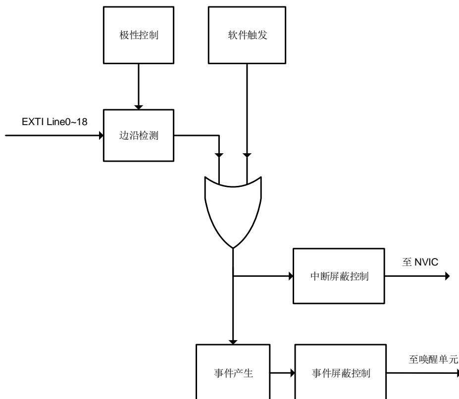
图 7-1. EXTI 框图
