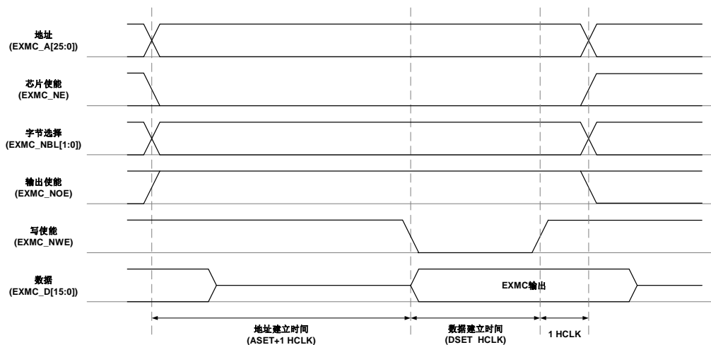
图 20-4. 模式 1 写访问
