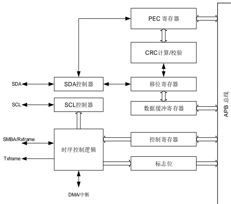
图 18-1. I2C 模块框图
