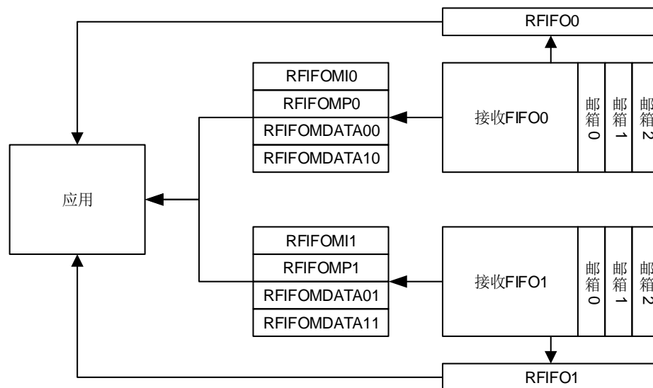
图 21-4. 接收寄存器
