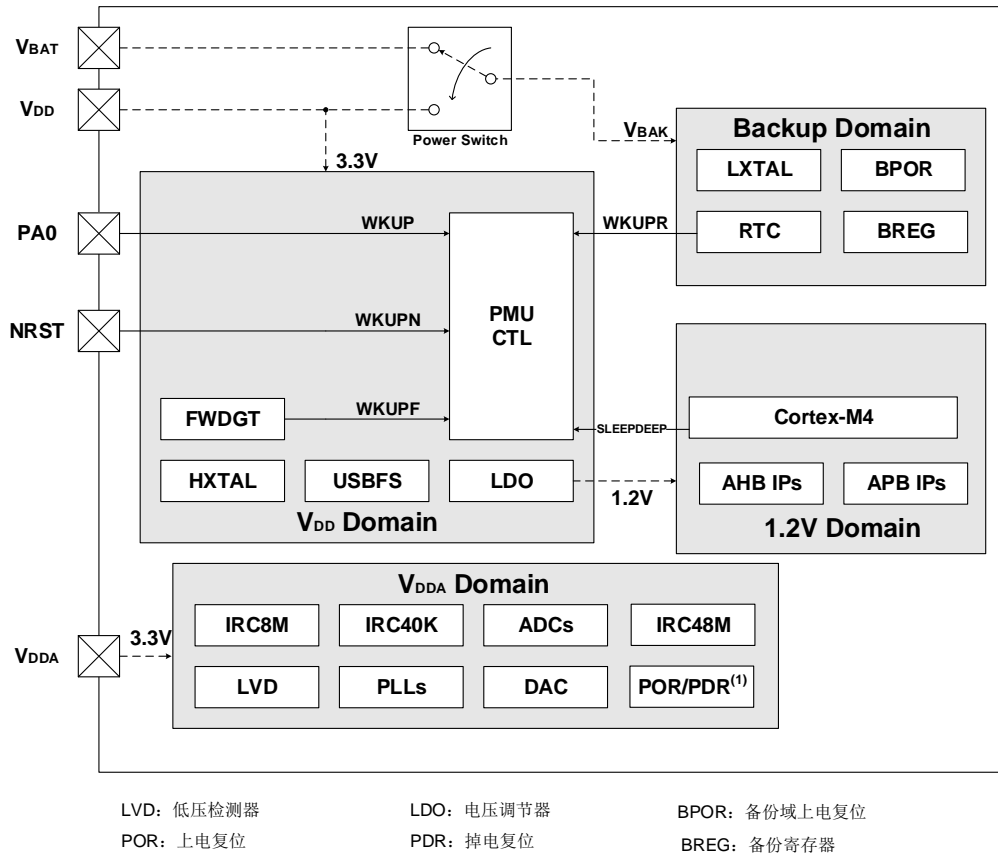
图3-1. 电源域概览
