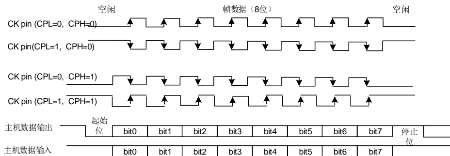
图 17-12. 8-bit 格式的 USART 同步通信波形 (CLEN=1)
