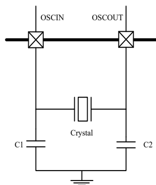
图5-3. HXTAL时钟源
