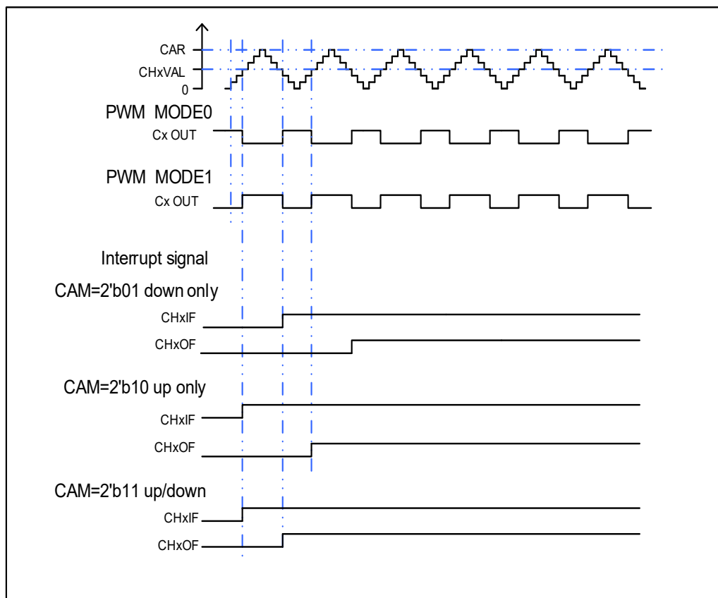
图 16-52. CAPWM 时序图
