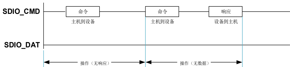
图 20-1. SDIO “无响应” 和 “无数据” 操作
