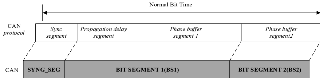
图 22-11. 位时序
