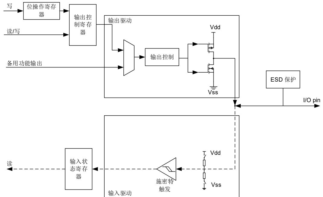
图 8-3. 输出配置
