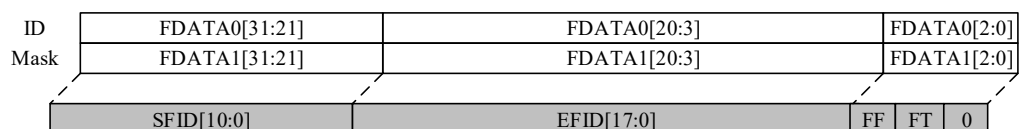
图 22-7. 32-bit 位宽掩码模式过滤器
