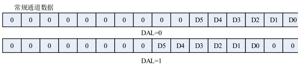
图 12-8. 6 位数据存储模式
