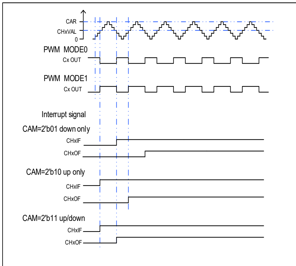
图 16-15. CAPWM 时序图
