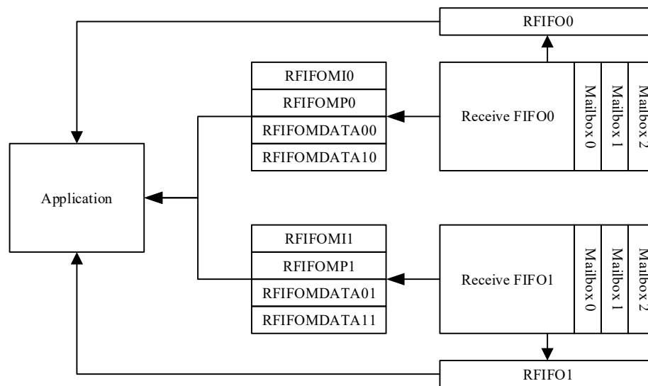
图 22-4. 接收寄存器
