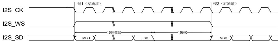
图 19-30. MSB 对齐标准时序图(DTLEN=00, CHLEN=1, CKPL=1)
