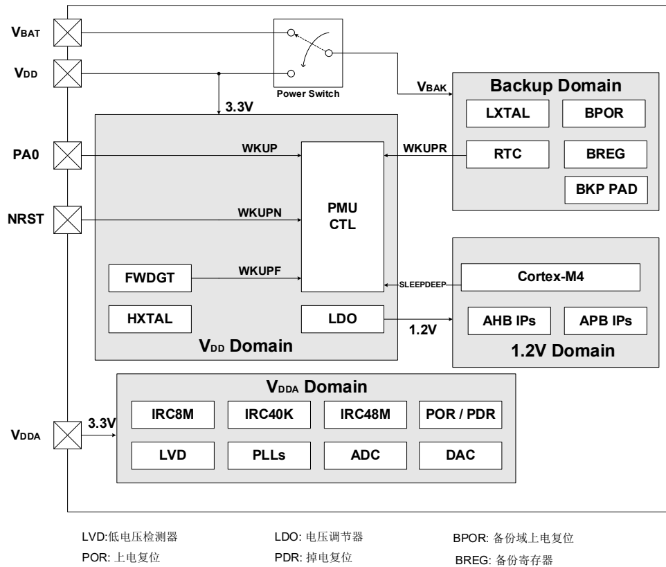
图3-1. 电源域概览
