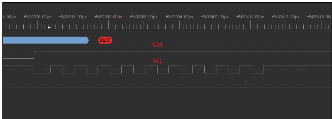
图 3-1. SCL 时钟信号释放总线测试
