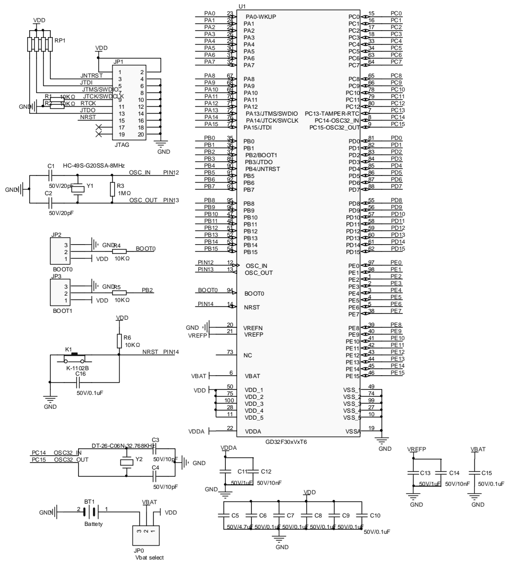
图 2-25. GD32F30x/GD32F403 推荐参考原理图设计
