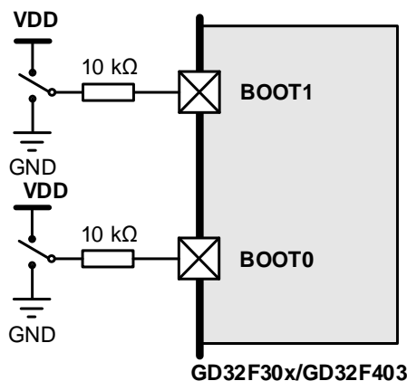
图 2-16. 推荐 BOOT 电路设计
