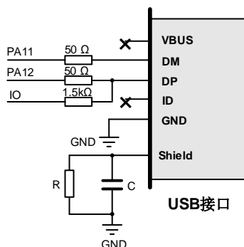
图 2-18. 推荐 USB-Device 参考电路
