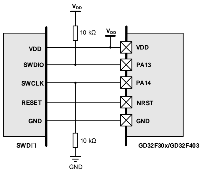
图 2-24. 推荐 SWD 接线参考设计
