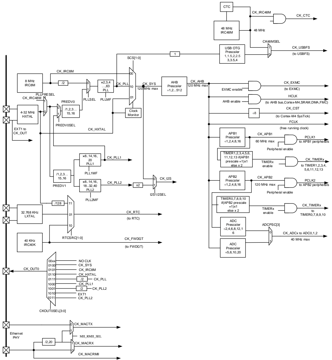
图 2-10. GD32F305xx & GD32F307xx 系列时钟树
