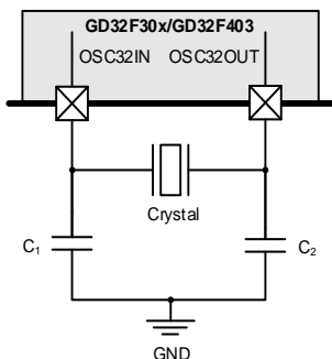
图 2-14. LXTAL 外部晶体电路
