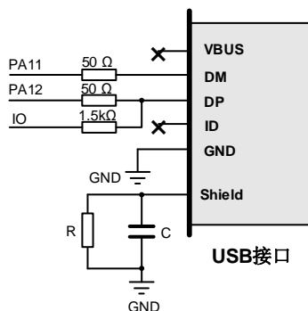
图 2-19. 推荐 USB-Device 参考电路
