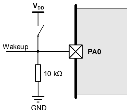
图 2-21. 推荐 Standby 外部唤醒引脚电路设计
