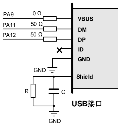
图 2-20. 推荐 USB-Device (USBFS) 参考电路
