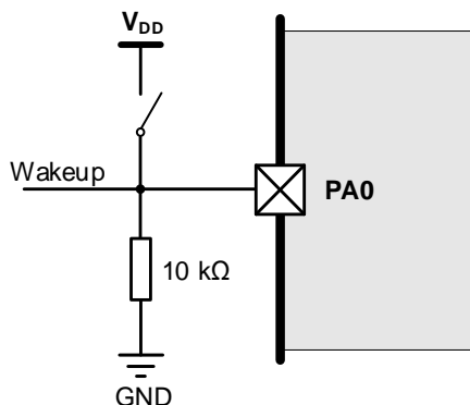
图 2-22. 推荐 Standby 外部唤醒引脚电路设计
