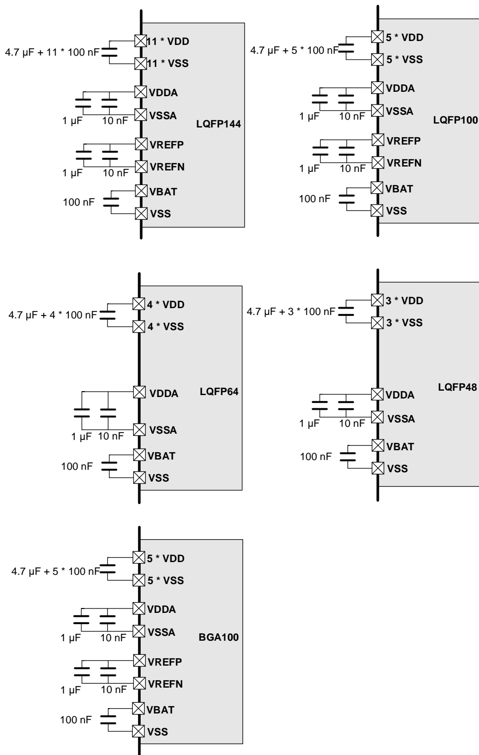
图 2-2. GD32F30x/GD32F403 系列推荐供电设计
