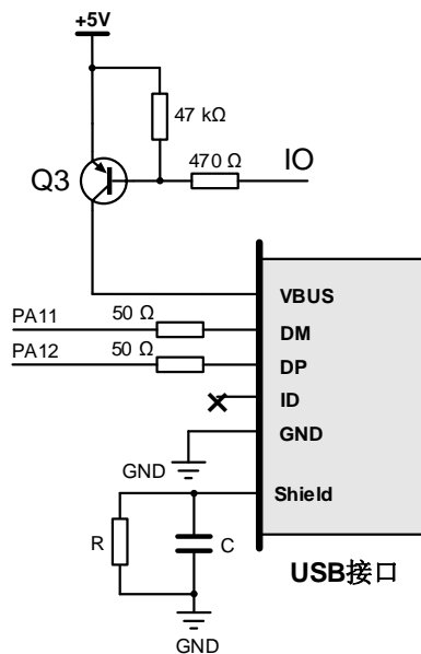
图 2-21. 推荐 USB-Host 参考电路
