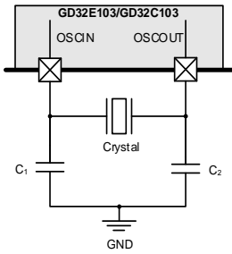
图 2-11. HXTAL 外部时钟电路
