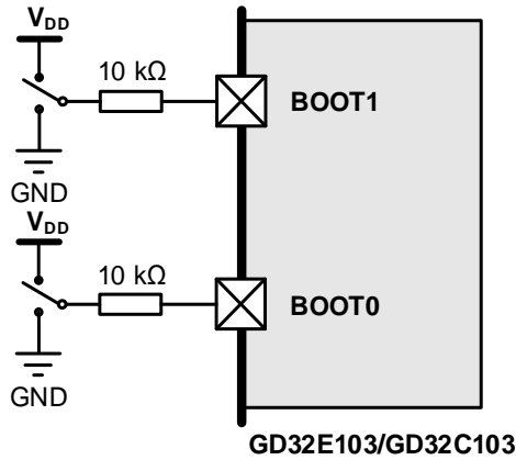
图 2-14. 推荐 BOOT 电路设计
