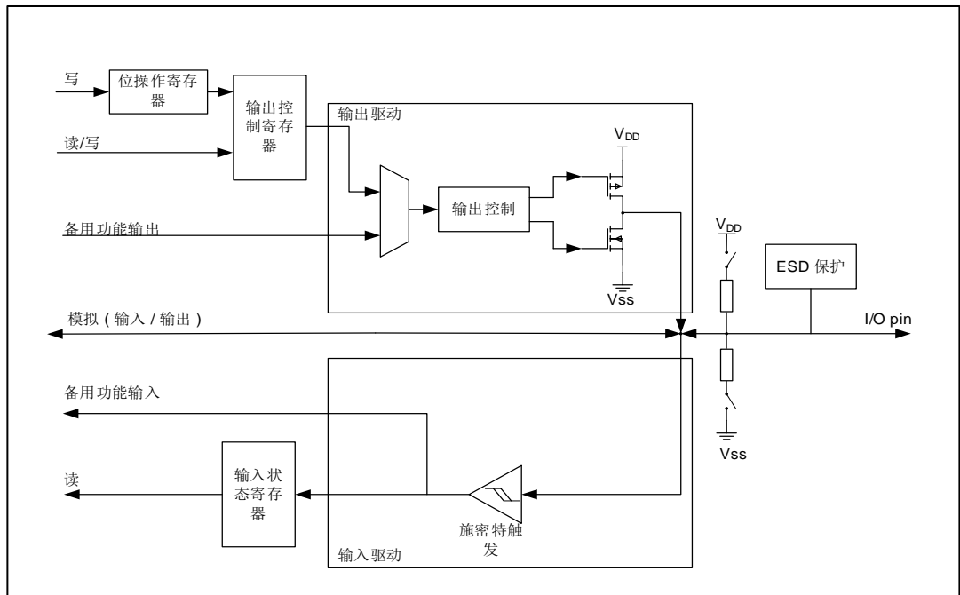
图 2-15. 标准 IO 的基本结构
