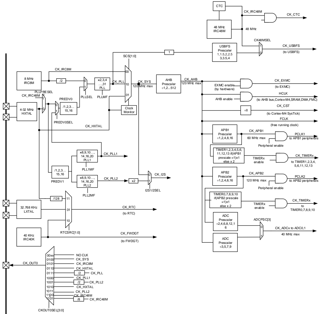
图 2-9. 时钟树
