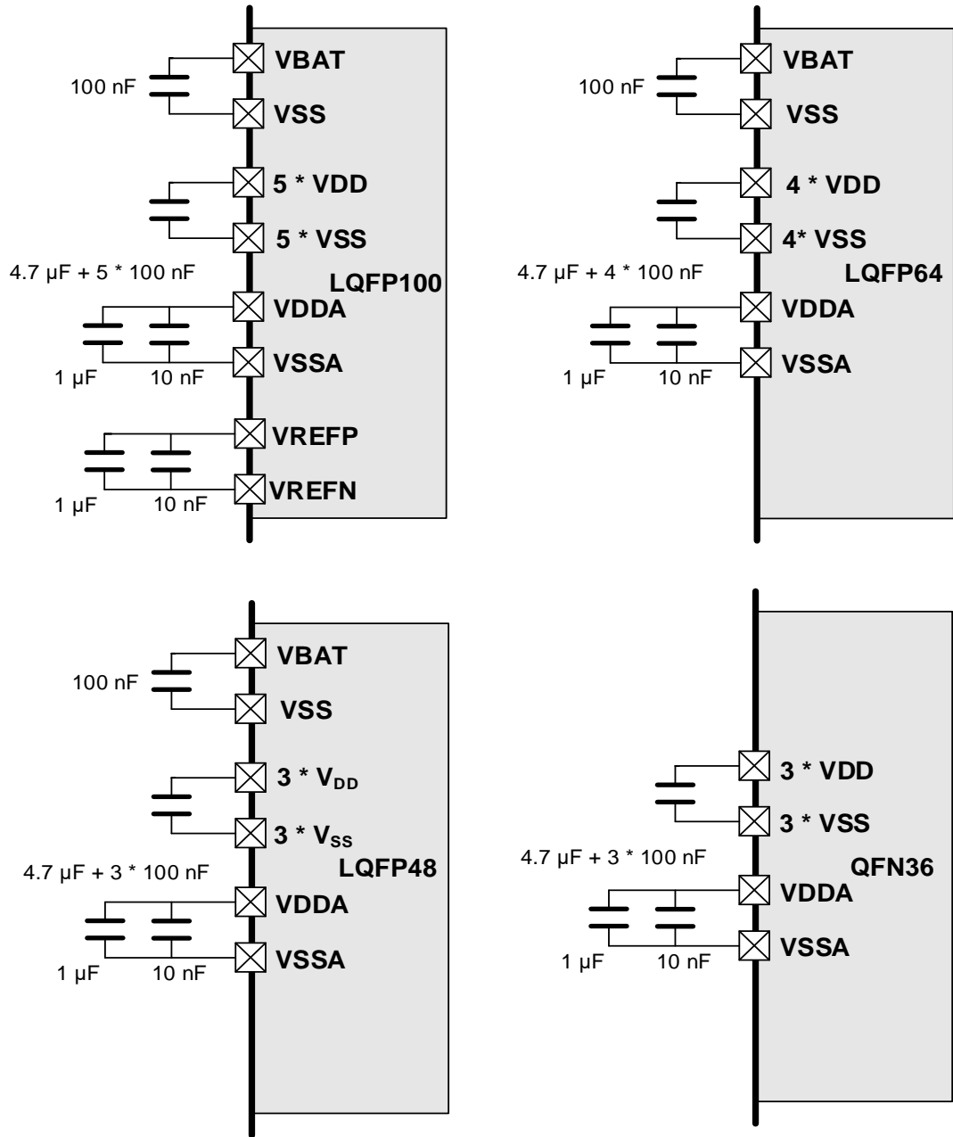
图 2-2. GD32E103/GD32C103 系列推荐供电设计
