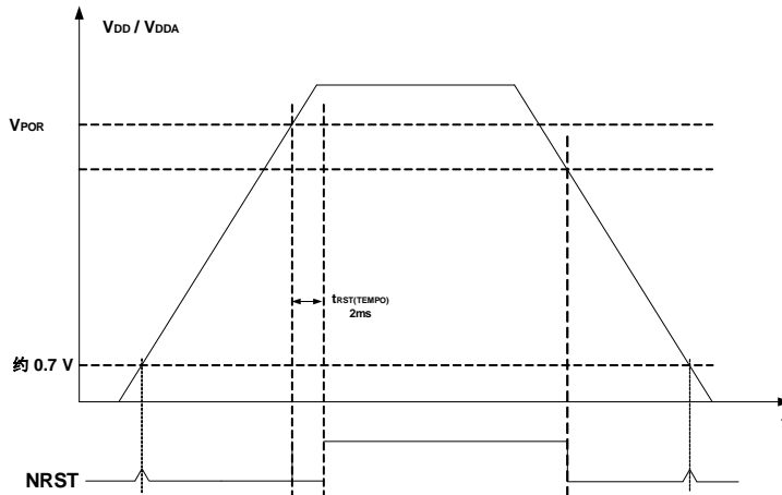
图 2-8. NRST 引脚上下电 MOS 管脉冲示意图
