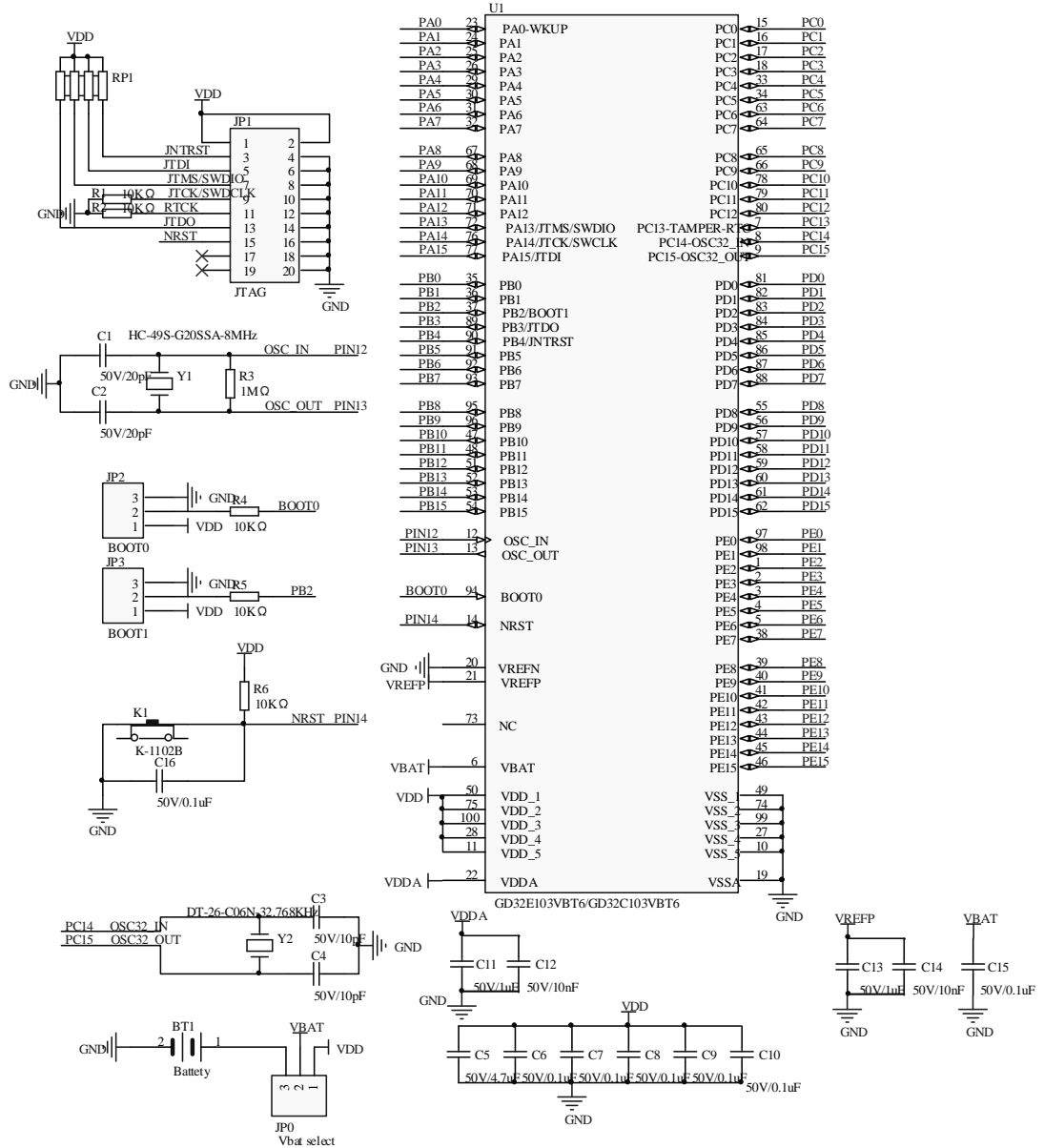
图 2-22. GD32E103/GD32C103 推荐参考原理图设计
