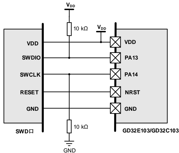
图 2-21. 推荐 SWD 接线参考设计
