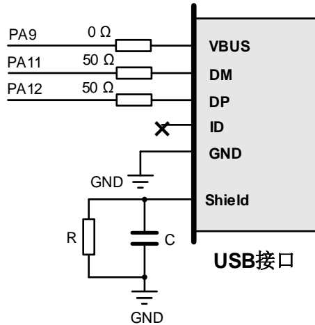
图 2-17. 推荐 USB-Device 参考电路
