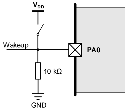
图 2-19. 推荐 Standby 外部唤醒引脚电路设计
