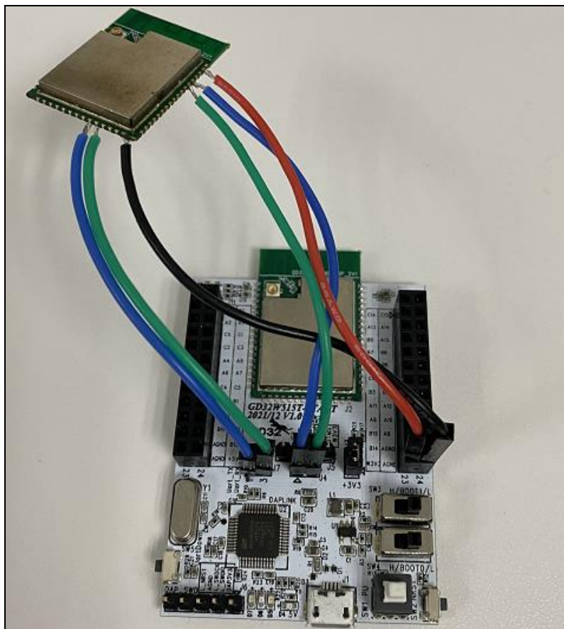
图 2-3. 单模组参考连接
