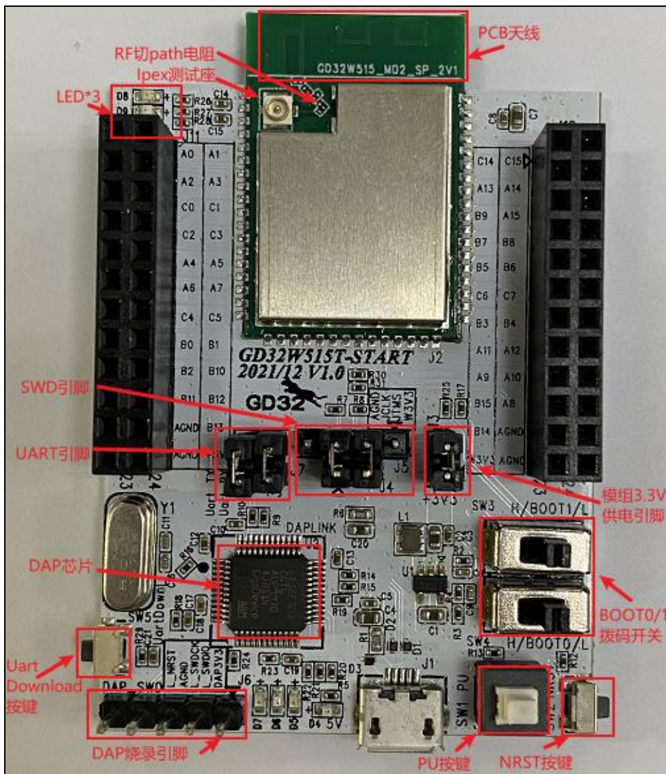
图 2-2. GD32 开发板参考连接
