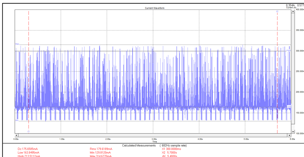
图 4-4. “UDP Rx”功耗
