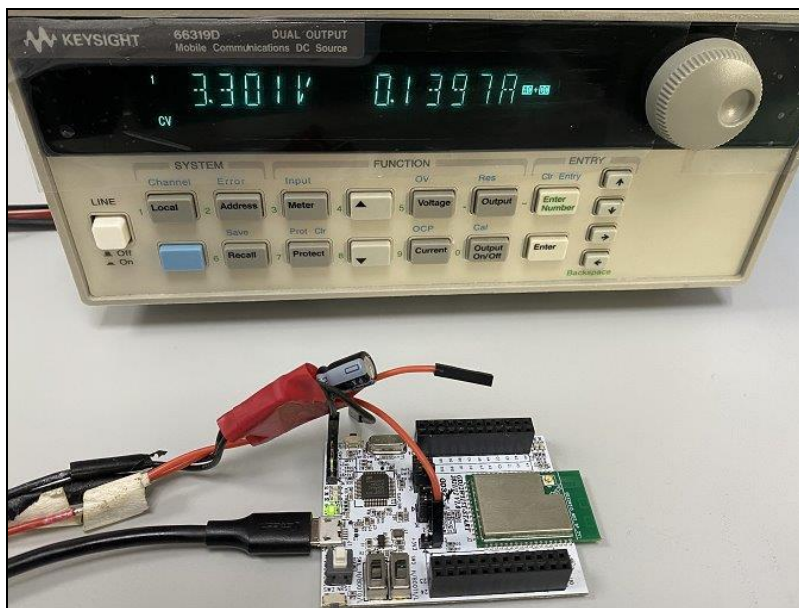
图 4-1. 功耗测试系统
