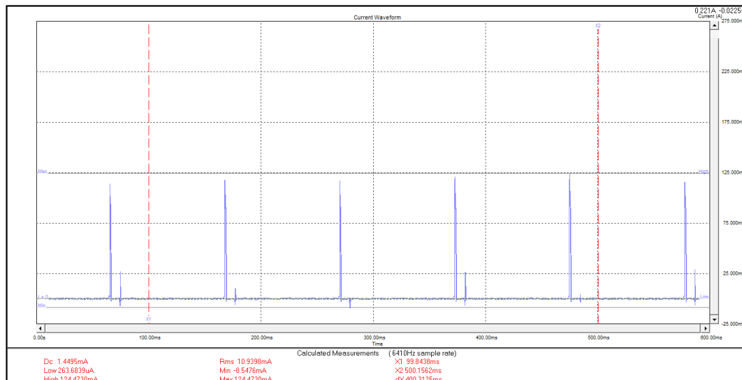
图 4-6. “DTIM = 1” 功耗
