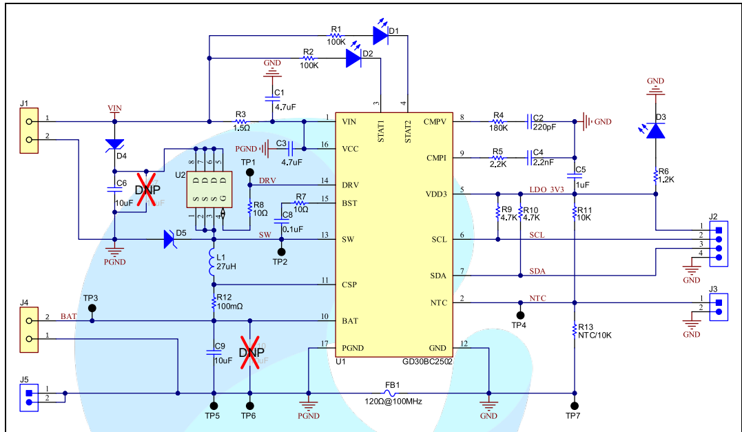
图 4-1. GD30BC2502-EVAL 板原理图
