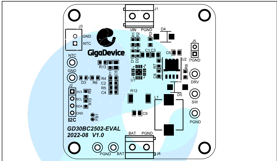
图 5-1. GD30BC2502-EVAL TopOverLay
