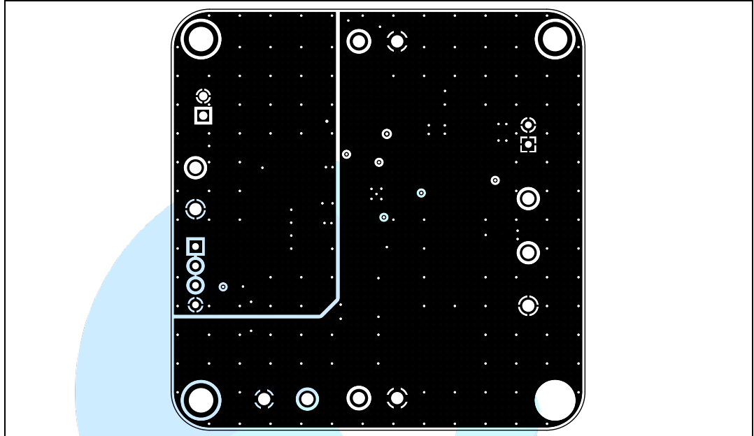
图 5-5. GD30BC2502-EVAL GND03
