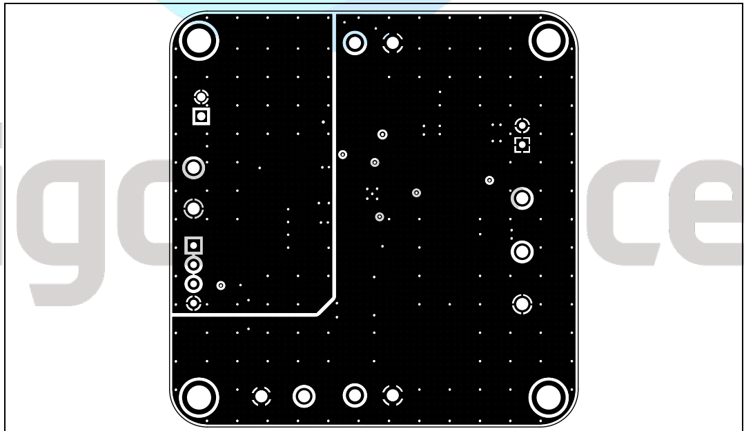
图 5-4. GD30BC2502-EVAL GND02
