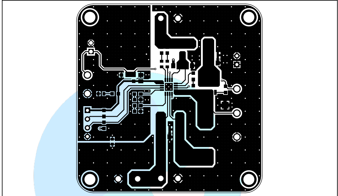
图 5-3. GD30BC2502-EVAL Top Layer
