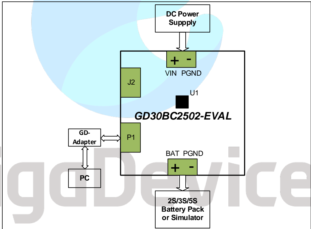
图 3-1. 硬件连接示意图
