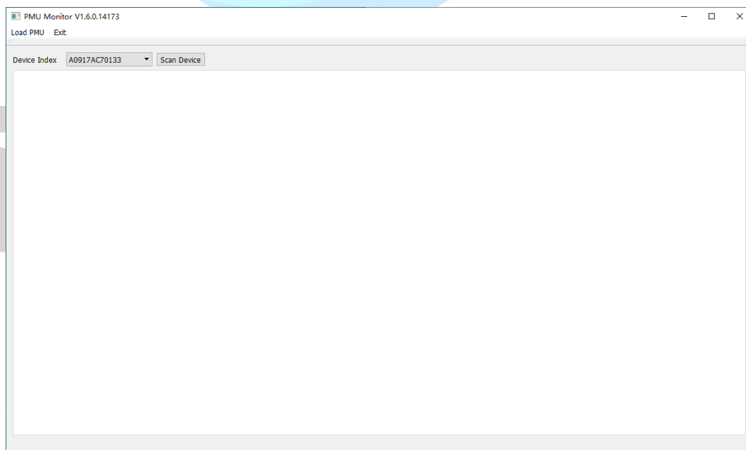
图 3-3. 软件界面
