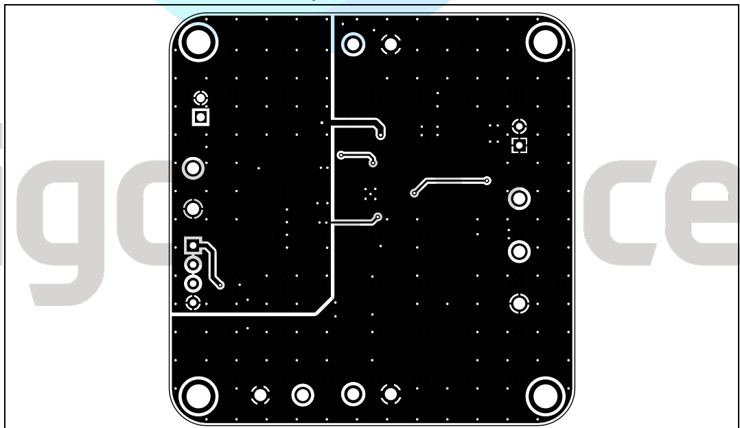
图 5-6. GD30BC2502-EVAL Bottom Layer
