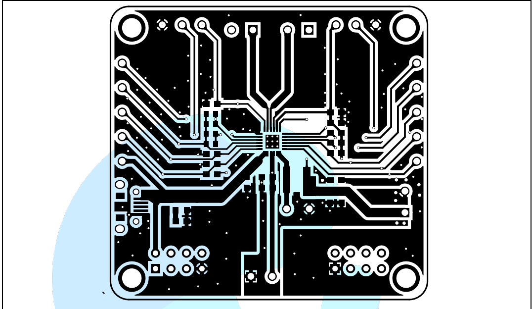
图 5-3. GD30WS8805 EVAL Top Layer
