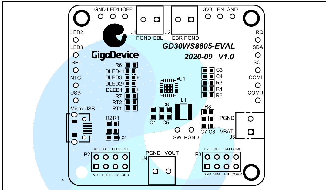
图 5-1. GD30WS8805 EVAL TOP Overlay
