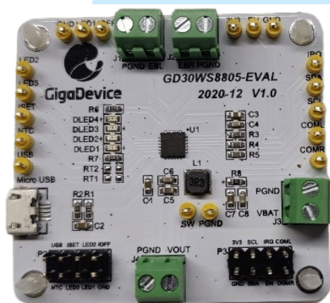
图 1-1. GD30WS8805 EVAL 板外观图
