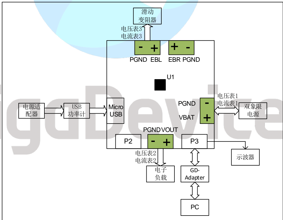
图 3-1. 硬件连接示意图
