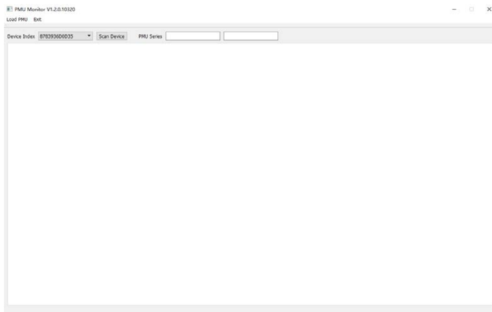
图 3-3. 软件界面
