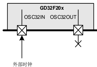
图 2-14. LXTAL 外部时钟电路
