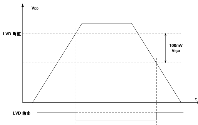
图2-5. LVD阈值波形图
