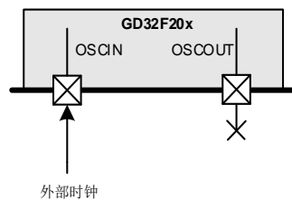
图 2-11. HXTAL 外部时钟电路
