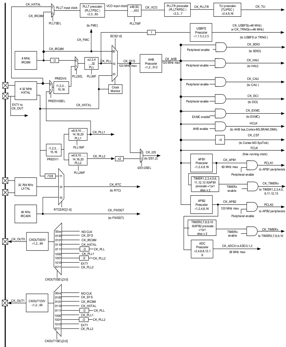
图 2-9. GD32F205x 系列时钟树
