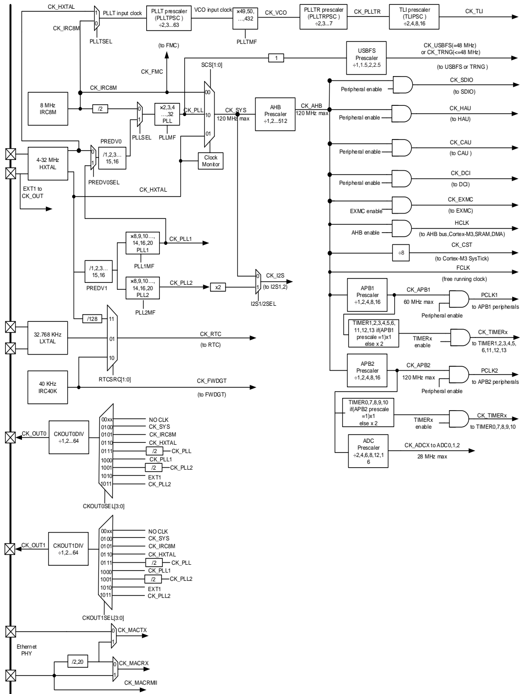
图 2-9. GD32F207x 系列时钟树
