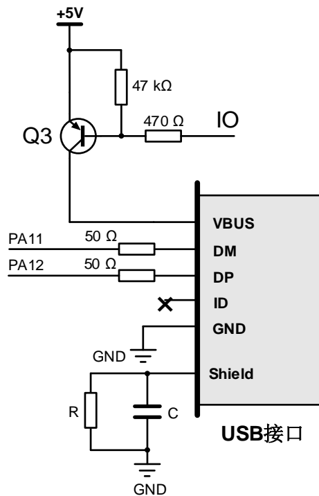
图 2-19. 推荐 USB-Host 参考电路
