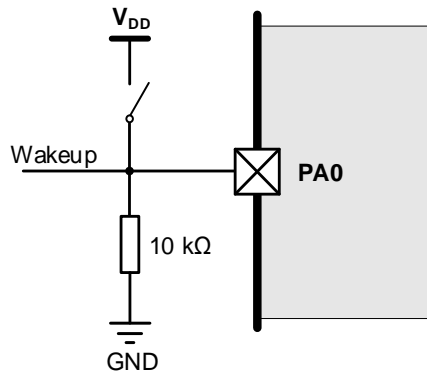
图 2-20. 推荐待机模式外部唤醒引脚电路设计
