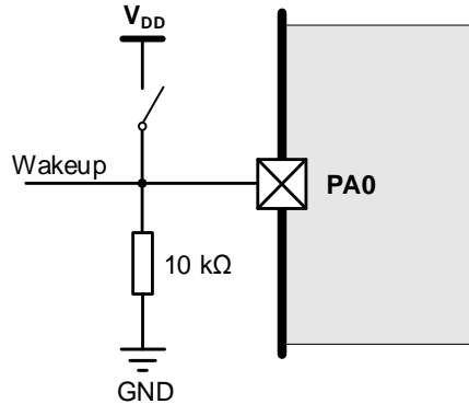
图 2-19. 推荐待机模式外部唤醒引脚电路设计
