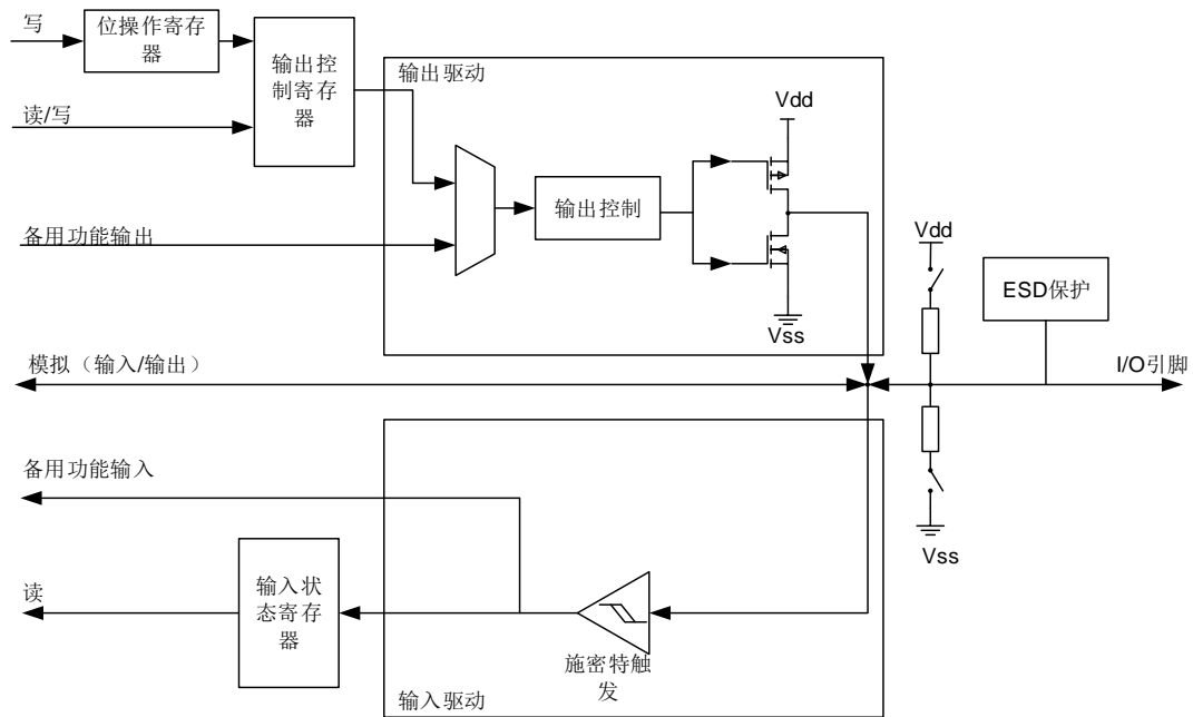
图 2-15. 标准 IO 的基本结构
