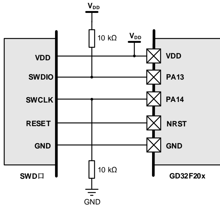
图 2-21. 推荐 SWD 接线参考设计
