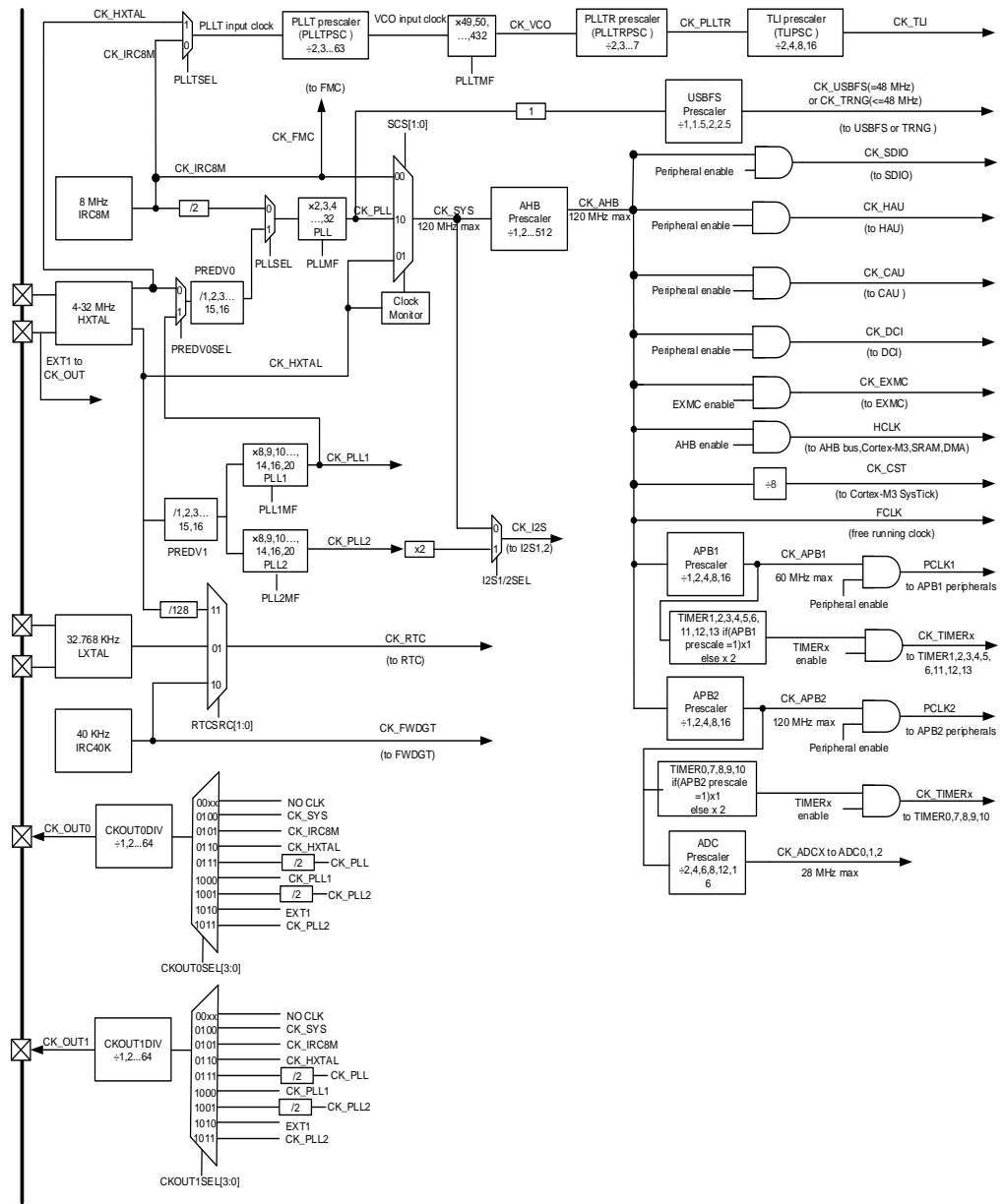
图 2-8. GD32F205x 系列时钟树
