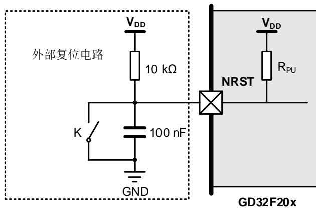
图 2-7. 推荐外部复位电路
