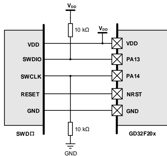
图 2-22. 推荐 SWD 接线参考设计
