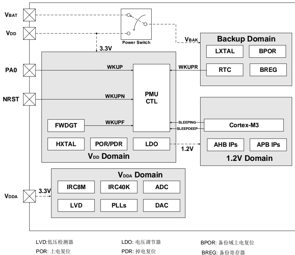
图 2-1. GD32F20x 系列电源域概览
