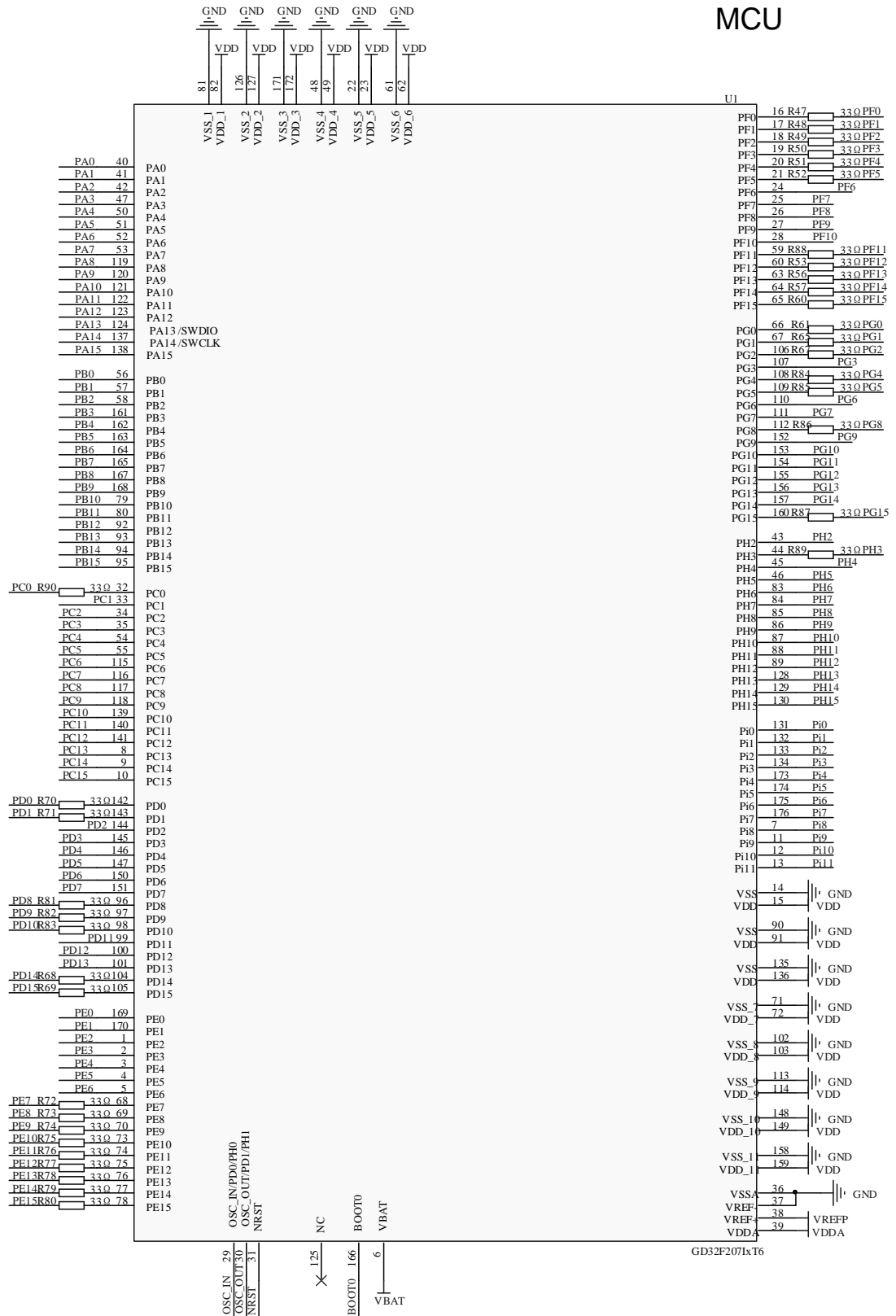
图 2-23. GD32F20x 系列推荐参考原理图设计
