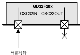
图 2-13. LXTAL 外部时钟电路
