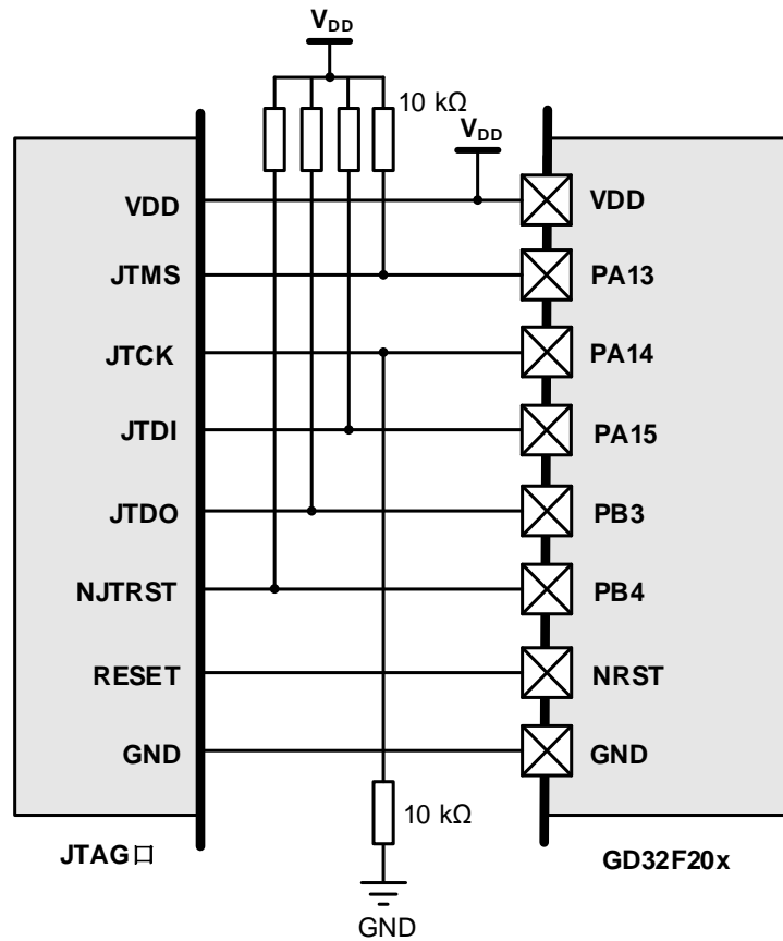
图 2-20. 推荐 JTAG 接线参考设计
