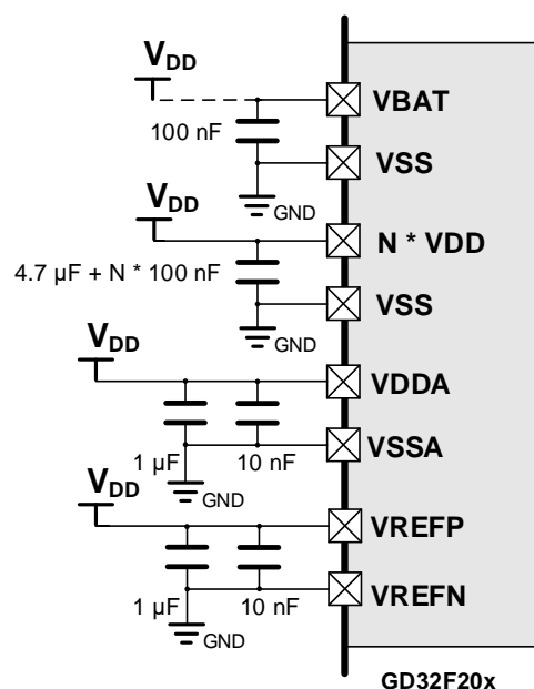
图 2-2. GD32F20x 系列推荐供电设计
