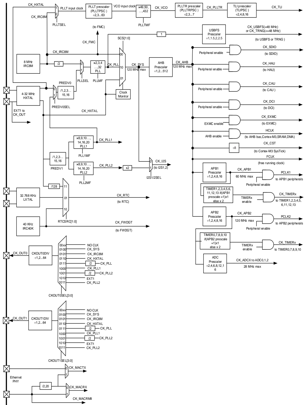
图 2-10. GD32F207x 系列时钟树
