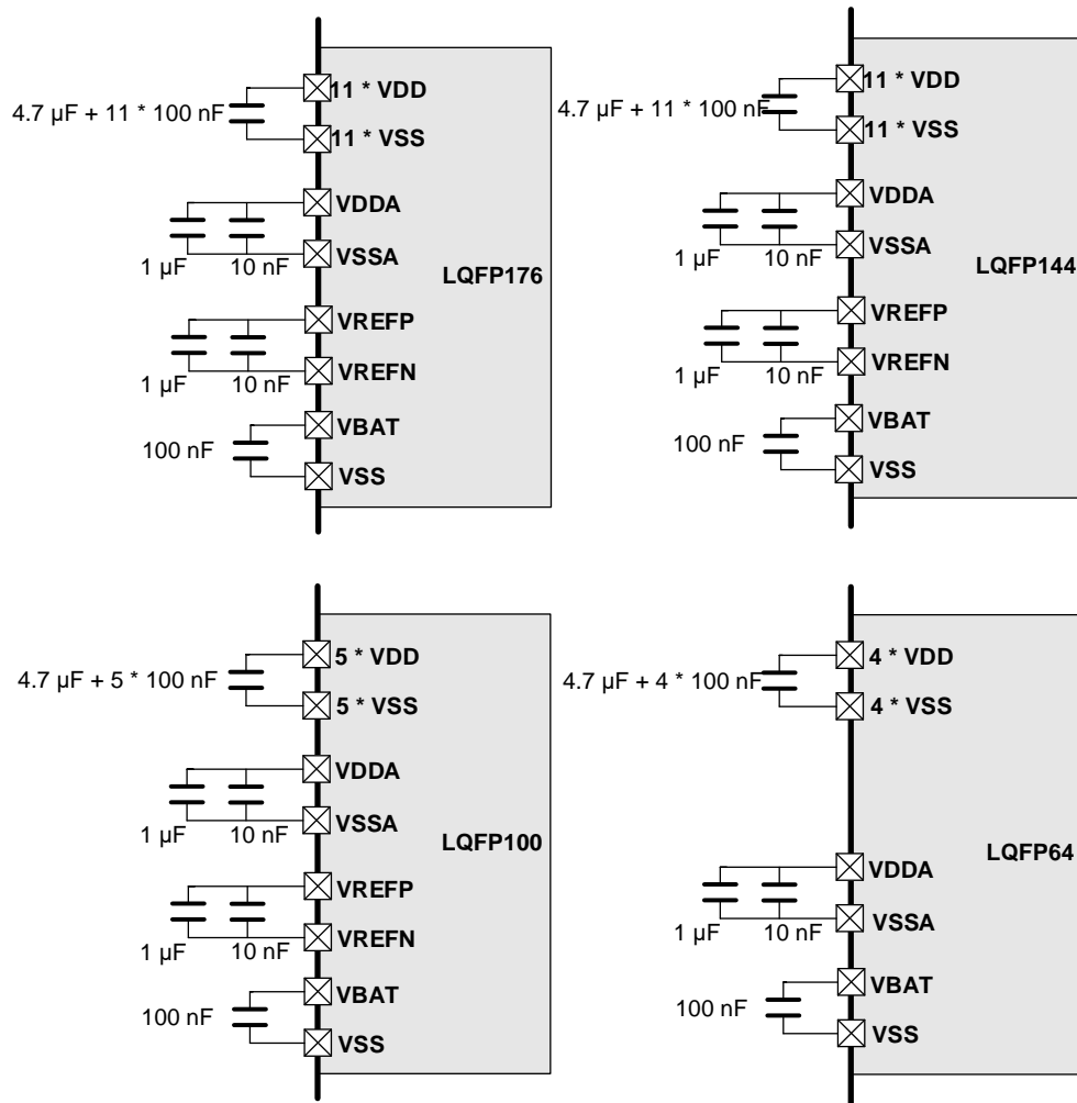
图 2-2. GD32F20x 系列推荐供电设计
