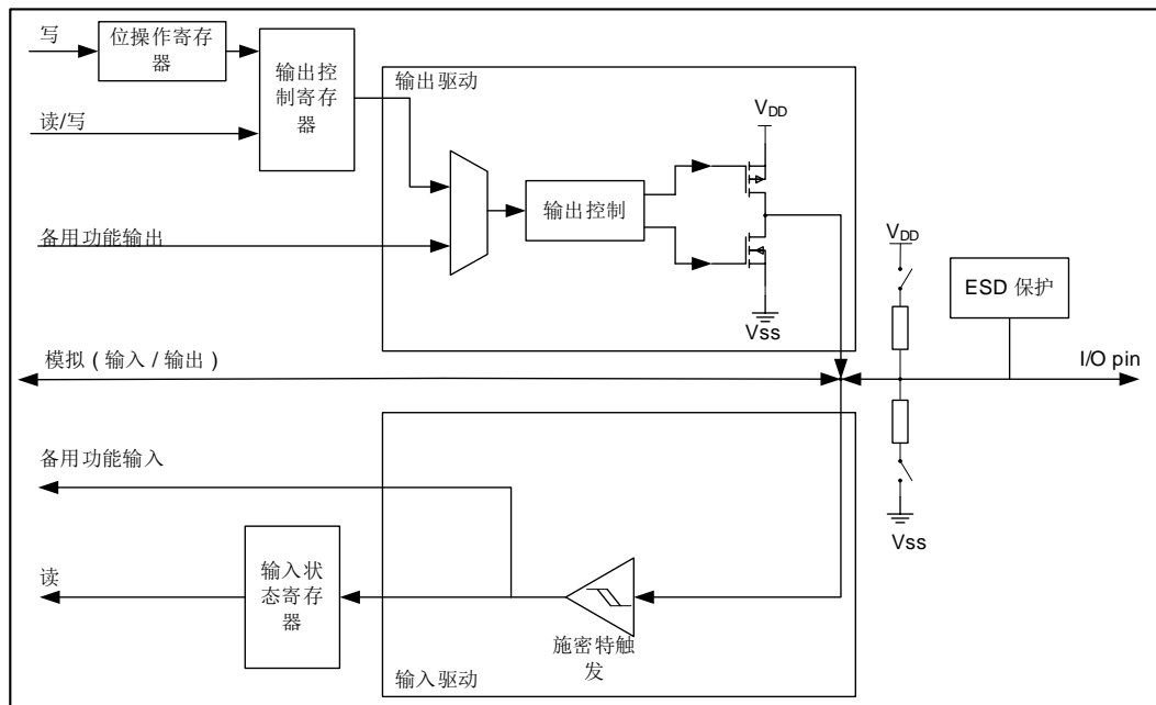
图 2-16. 标准 IO 的基本结构
