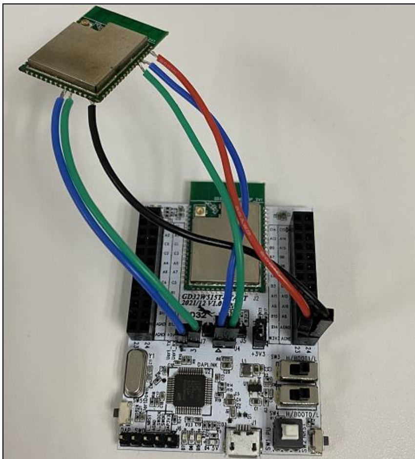
图 2-3. 单模组参考连接
