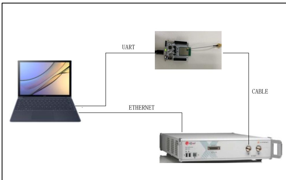
图 2-1. RF 测试系统
