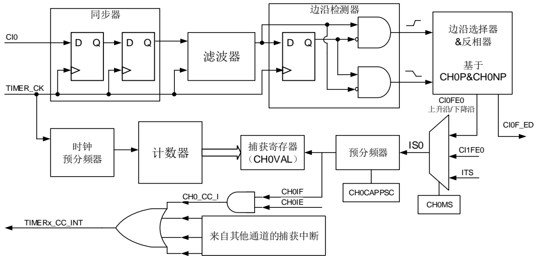
图 24-58. 输入捕获逻辑
