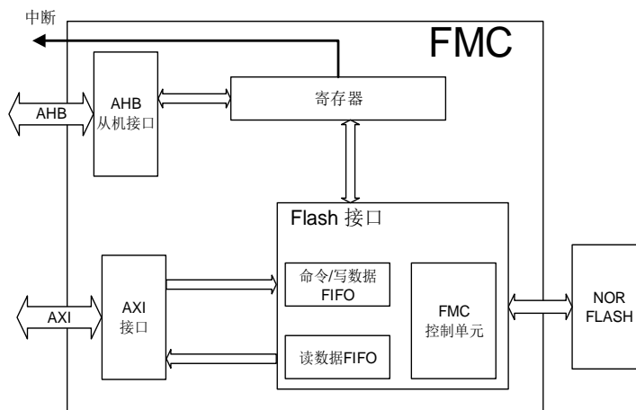
图 3-1. FMC 框图
