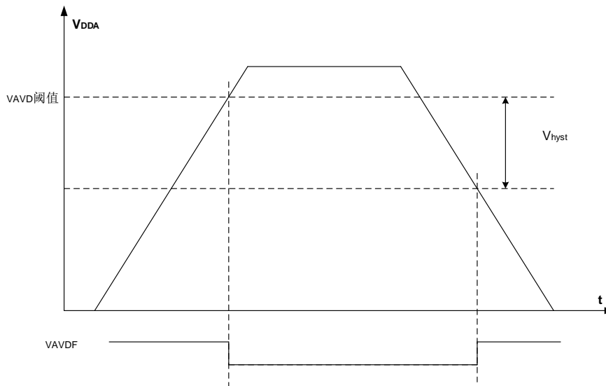
图 5-6. VAVD 阈值监测波形图
