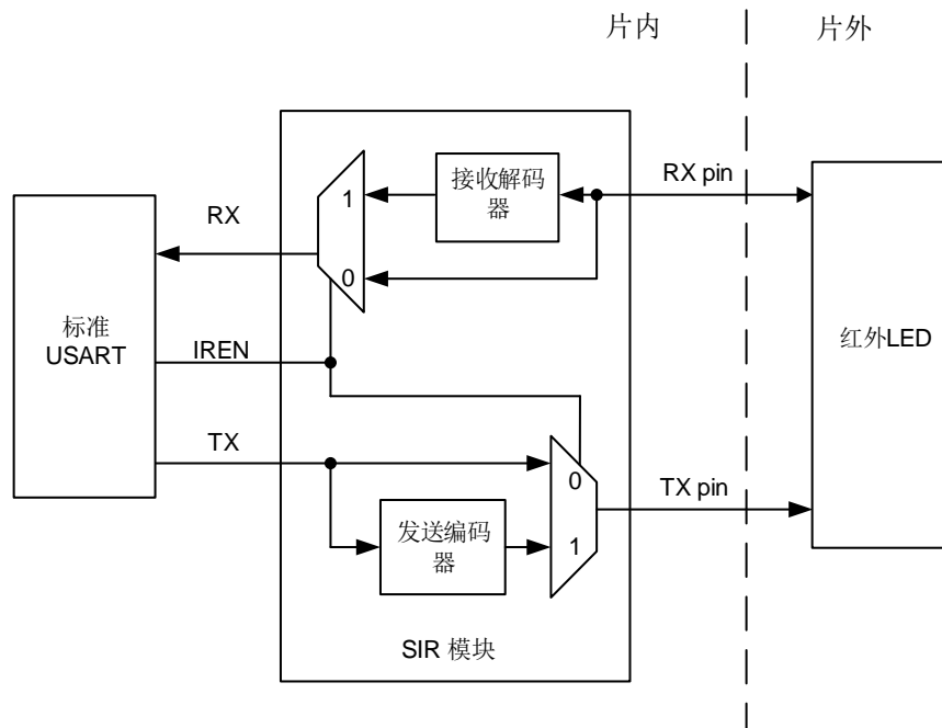
图 25-13. IrDA SIR ENDEC 模块
