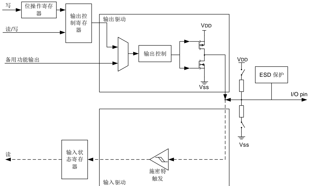
图 10-3. 输出配置
