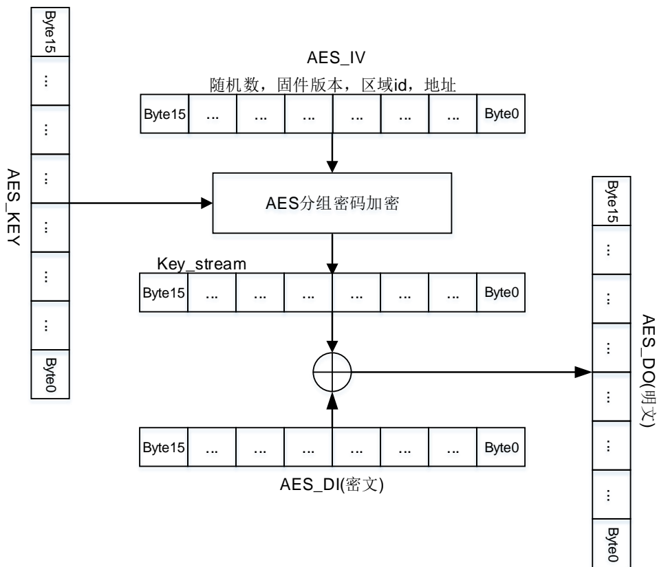
图 46-2. CTR 下的 AES-128 解密流
