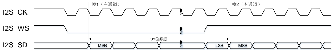
图 27-23. I2S 飞利浦标准时序图 (DTLEN = 10, CHLEN = 1, CKPL = 1)
