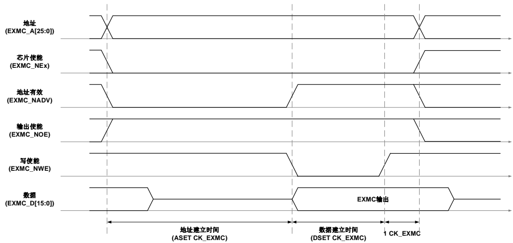
图 38-13. 模式 B 写时序
