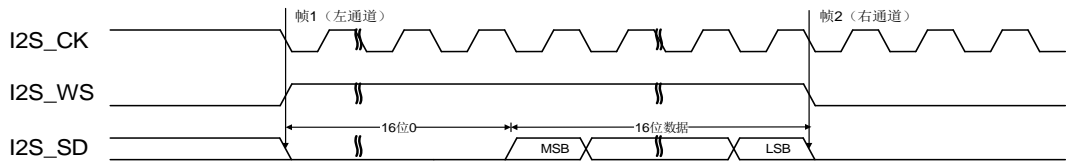
图 27-39. LSB 对齐标准时序图 (DTLEN = 00, CHLEN = 1, CKPL = 1)
