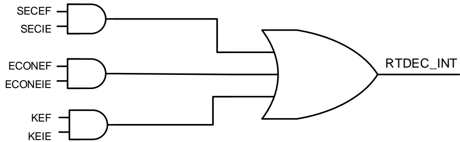
图 46-3. RTDEC 中断框图
