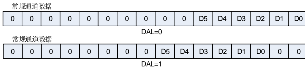
图 20-9. 6 位数据存储模式
