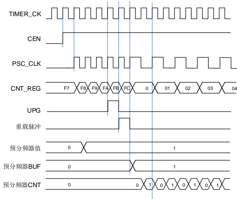
图 24-128. 当预分频器的参数从 1 变到 2 时，计数器的时序图
