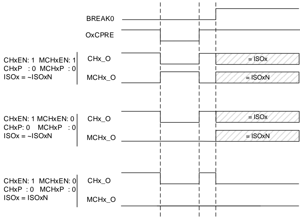
图 24-123. 通道响应 BREAK0 中止输入（高电平有效）时，输出信号的行为（IOS=1）
