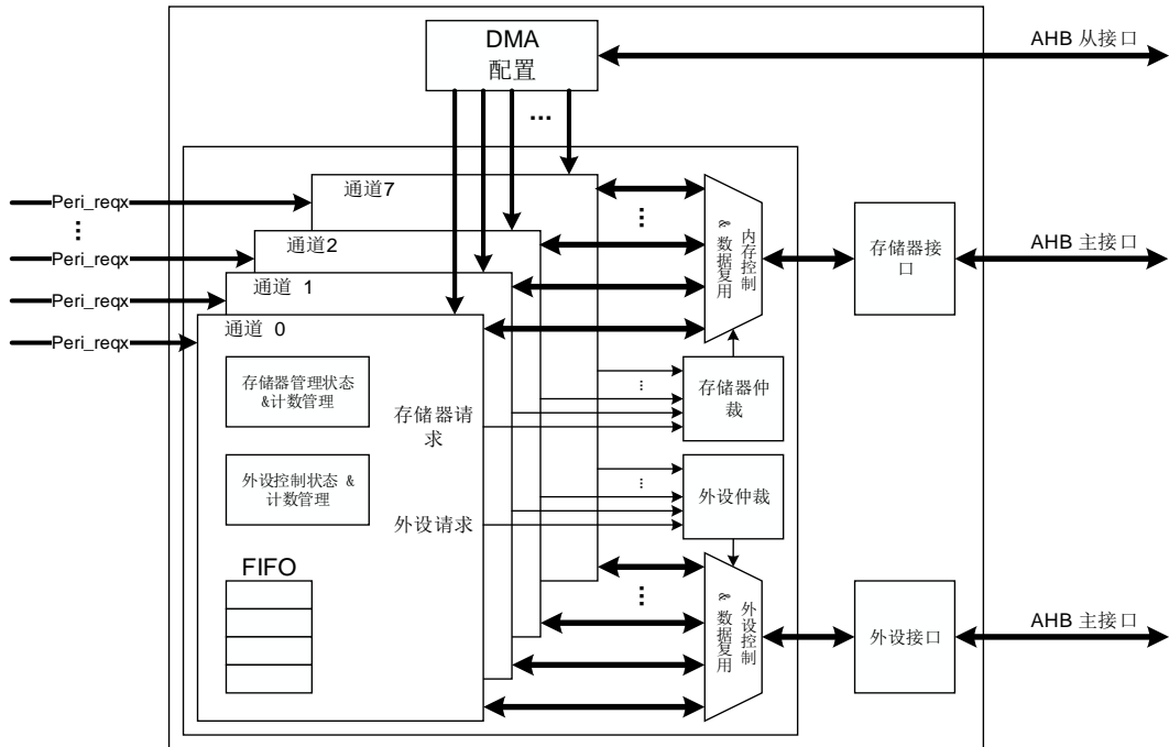
图 16-1. 系统架构
