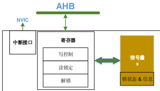
图 48-1. HWSEM 框图
