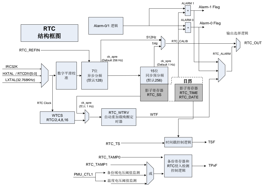
图 23-1. RTC 结构框图
