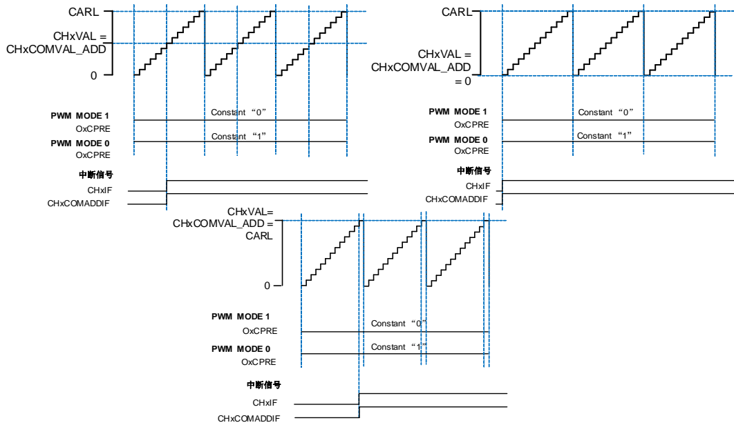
图 24-95. 通道 x 输出 PWM (CHxVAL = CHxCOMVAL_ADD)
