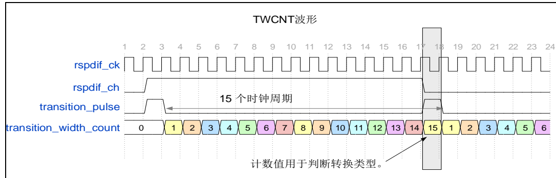
图 33-6. TWCNT 波形
