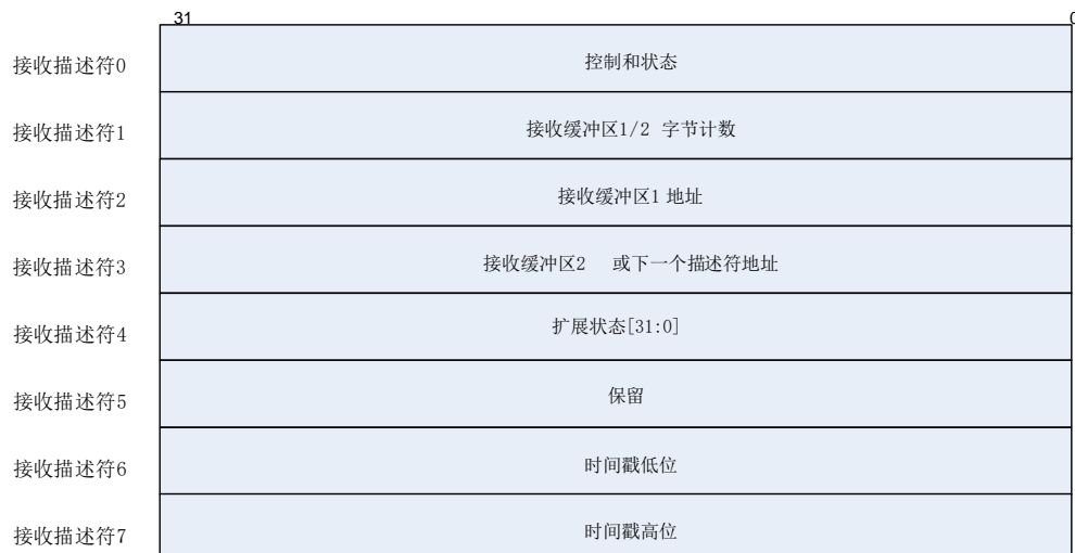
图 43-10. 增强接收描述符
