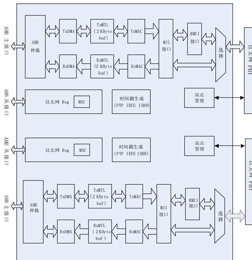
图 43-1. 以太网模块框图
