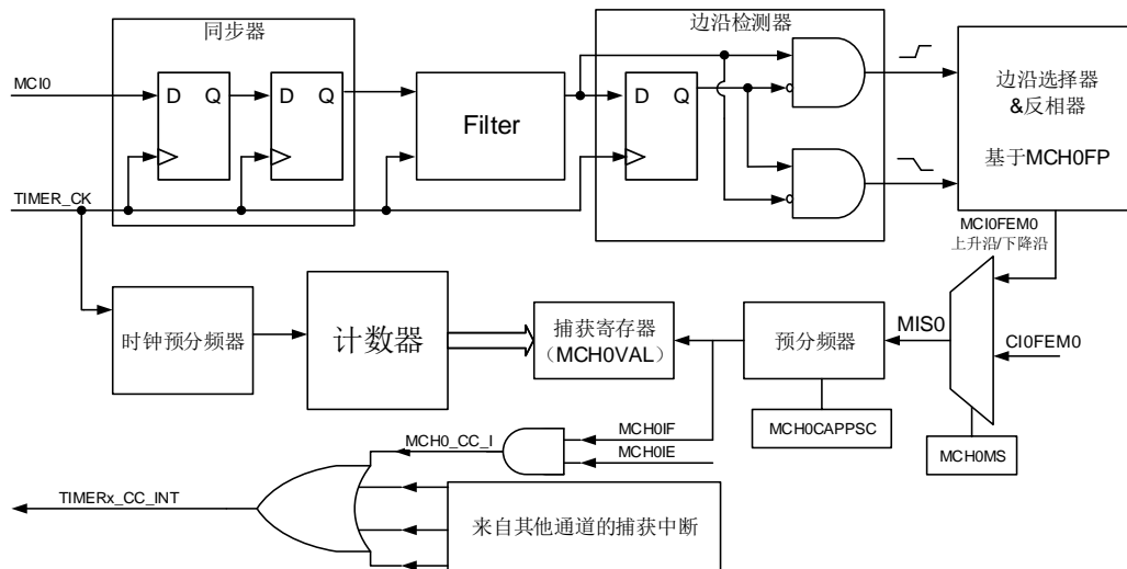
图 24-116. 多模式通道 0 输入捕获逻辑
