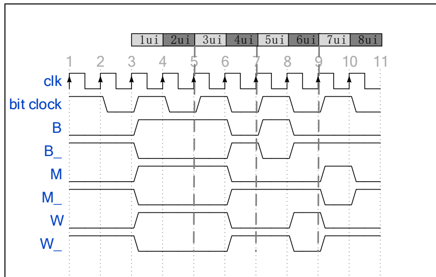
图 33-4. S/PDIF 报头
