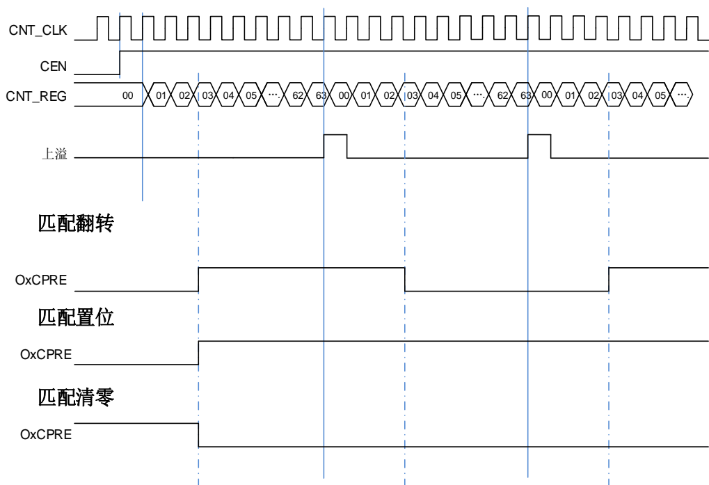
图 24-92. 三种输出比较模式
