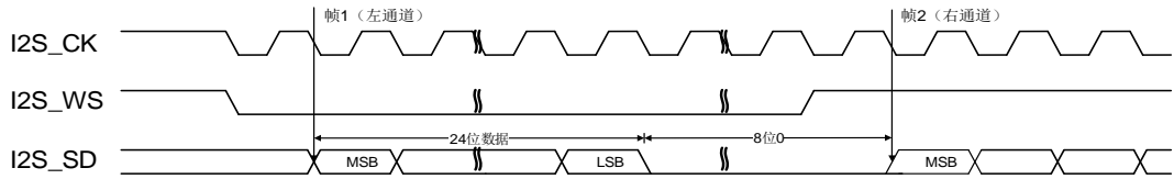
图 27-25. I2S 飞利浦标准时序图 (DTLEN = 01, CHLEN = 1, CKPL = 1)
