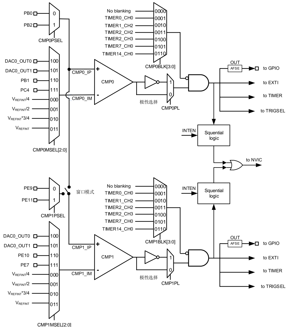
图 44-1. 比较器框图
