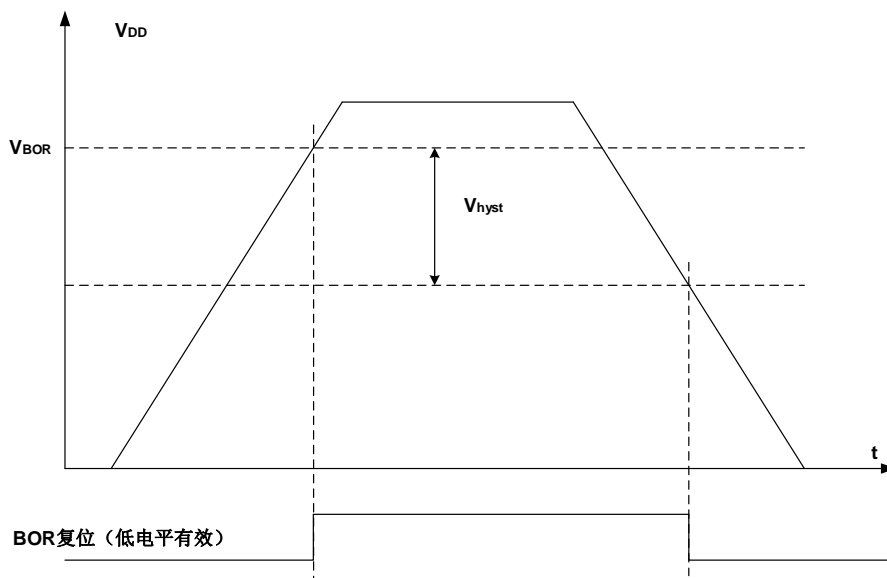
图5-4. BOR波形图
