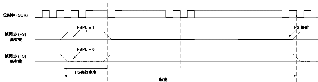
图 34-4. FS 极性
