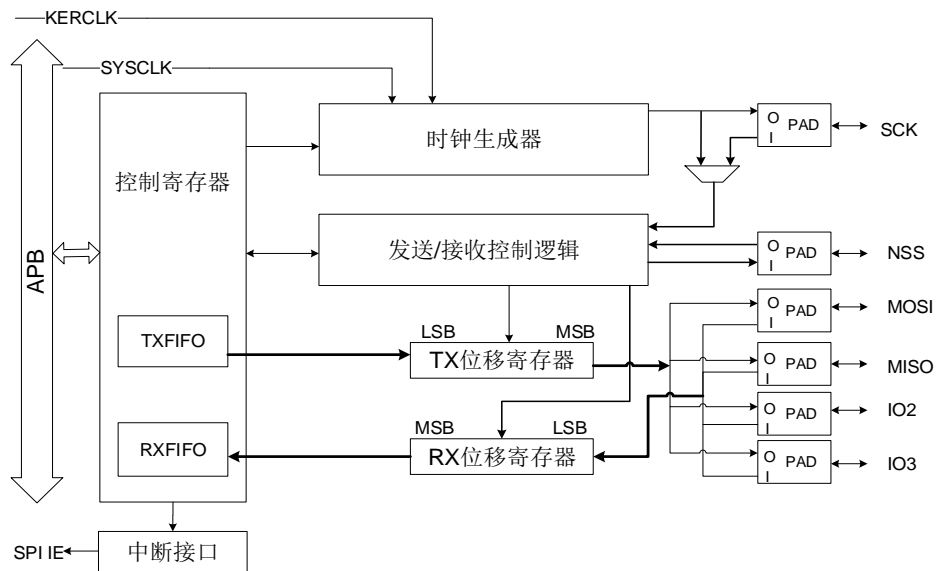
图 27-1. SPI 结构框图
