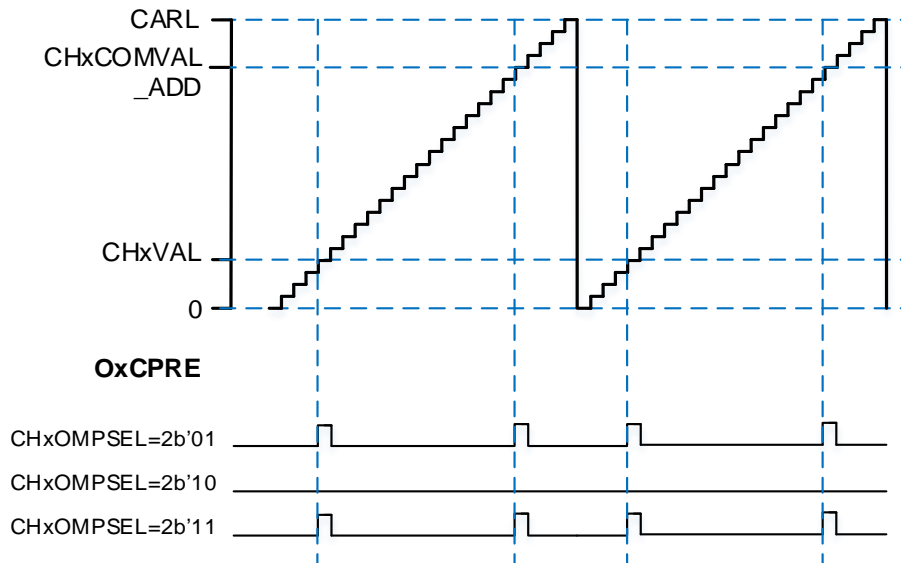
图 24-25. 边沿对齐模式下 CHx_O 输出脉冲 ( CHxOMPSEL \neq 2'b00 )
