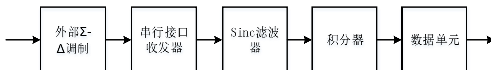
图 45-7. HPDF 模块外部输入数据处理流程
