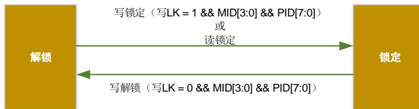
图 48-2. HWSEM 状态机
