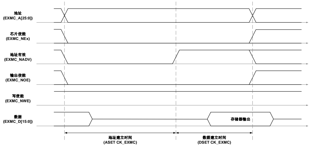
图 38-12. 模式 2 写时序
