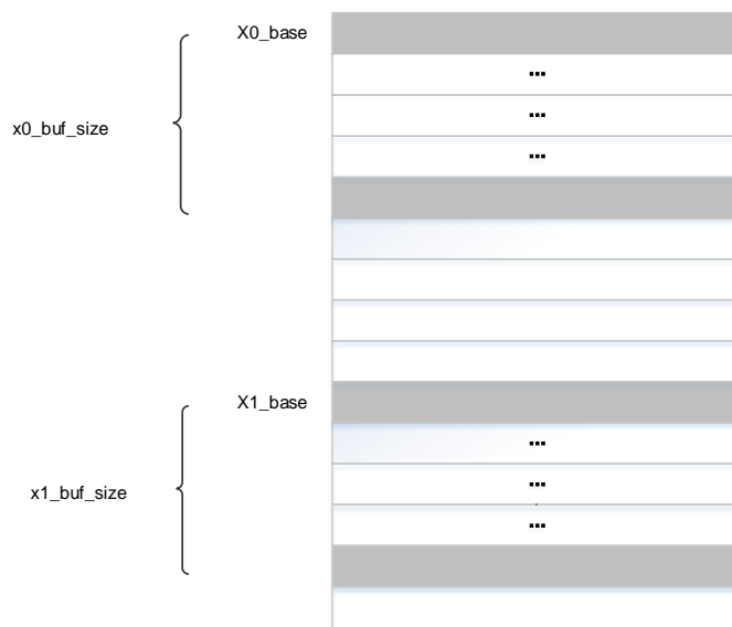
图 47-2. 输入缓冲区
