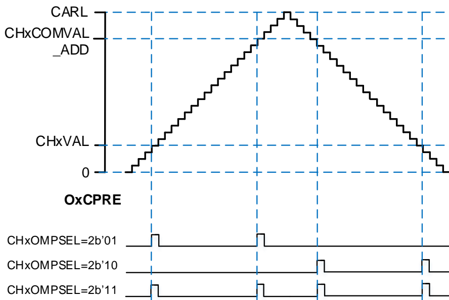
图 24-26. 中央对齐模式下 CHx_O 输出脉冲 ( CHxOMPSEL \neq 2'b00 )
