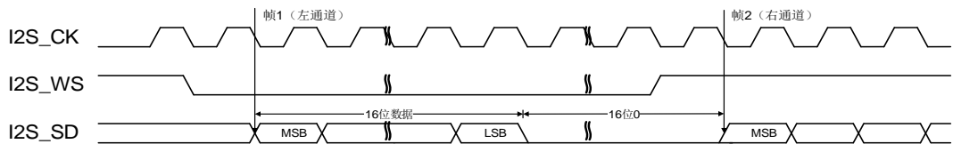
图 27-26. I2S 飞利浦标准时序图 (DTLEN = 00, CHLEN = 1, CKPL = 0)
