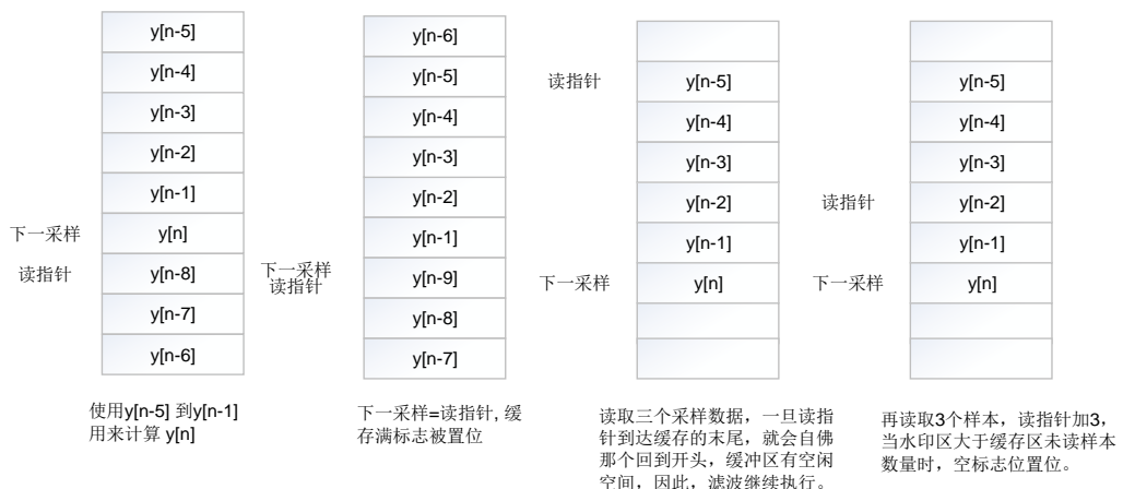
图 47-6. 循环输出缓冲区区域
