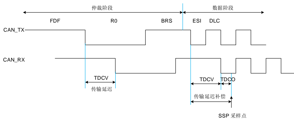
图 42-2. 传输延迟
