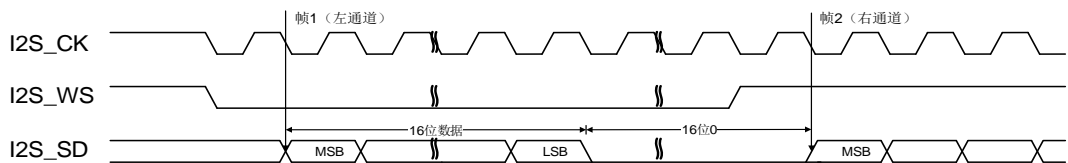
图 27-27. I2S 飞利浦标准时序图 (DTLEN = 00, CHLEN = 1, CKPL = 1)
