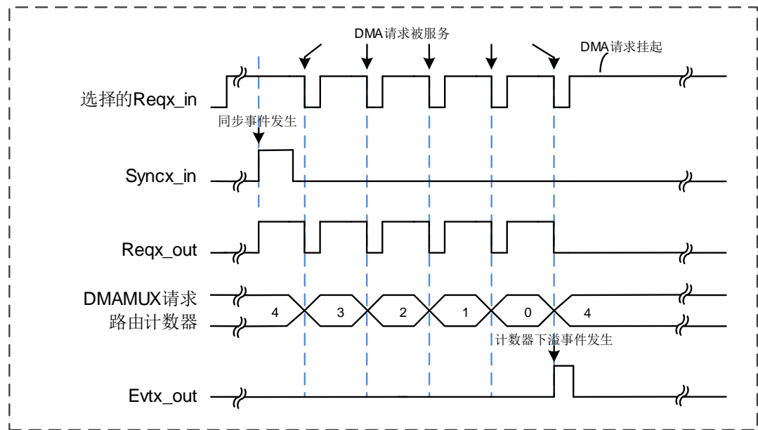
图 18-2. 同步模式
