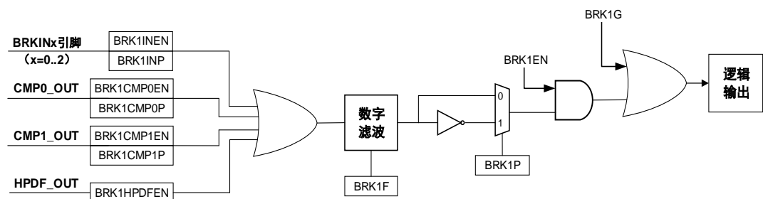
图 24-29. BREAK1 中止功能逻辑图
