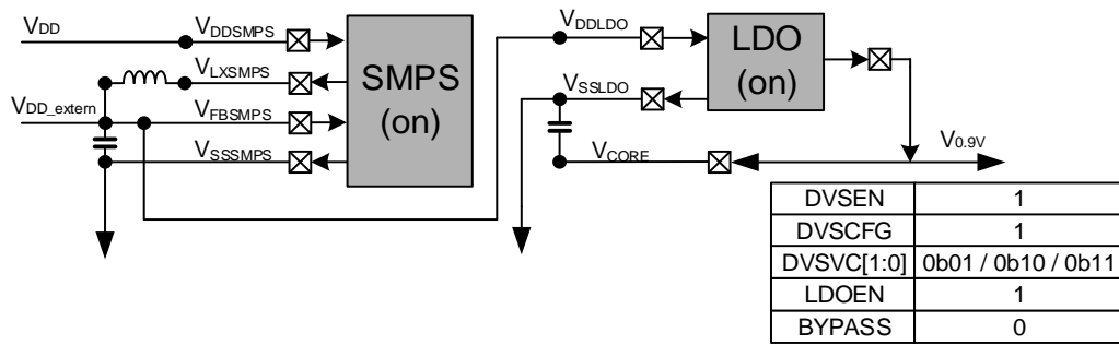
SMPS为LDO和外部供电，LDO供电V0.9V电源域
