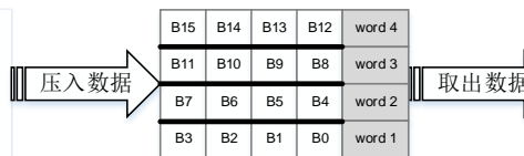
图 16-4. PWIDTH 为‘00’时，数据的打包/解包
