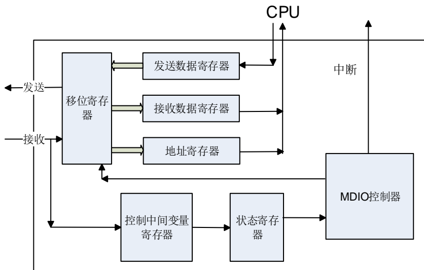
图37-2. MDIO框图
