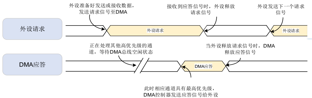
图 16-3. 握手机制
