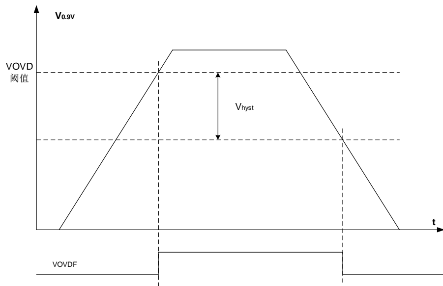
图 5-14. VOVD 波形
