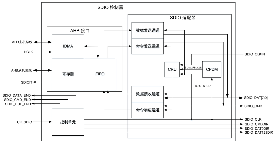
图 36-6. SDIO 框图
