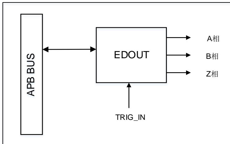
图 41-1. EDOUT 模块结构框图
