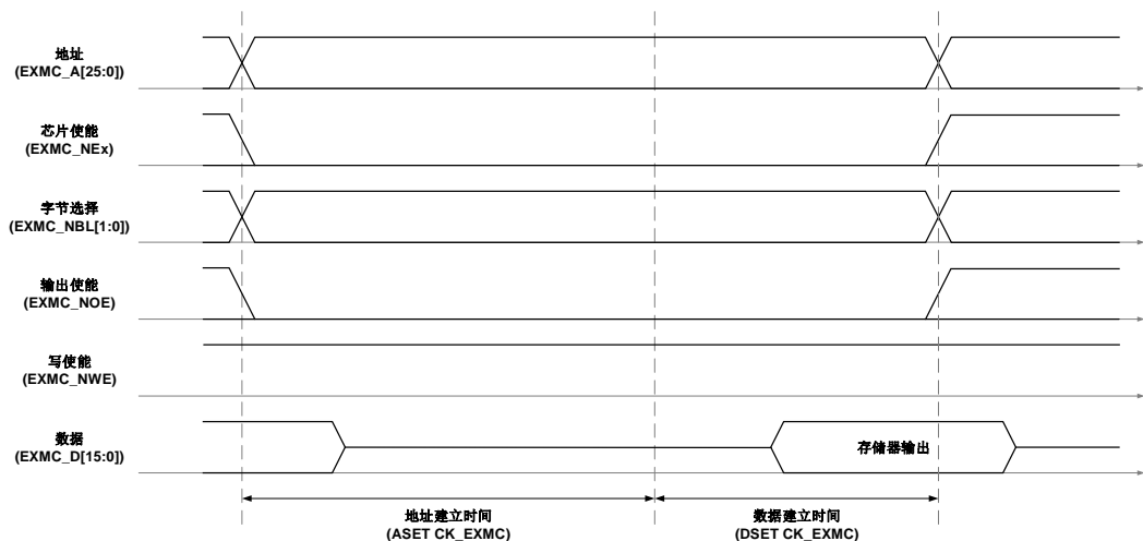
图 38-7. 模式 1 读时序
