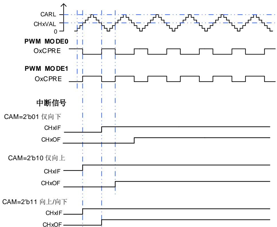
图 24-62. CAPWM 时序图
