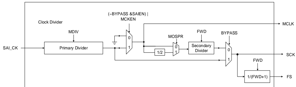
图 34-2. 时钟分频逻辑
