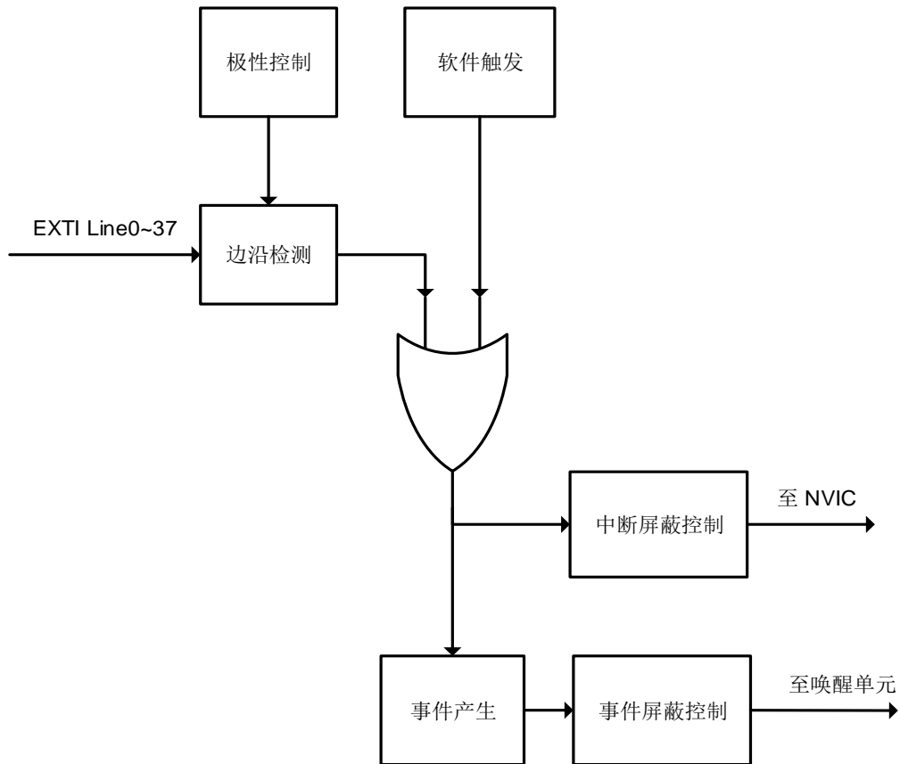
图 8-1. EXTI 框图
