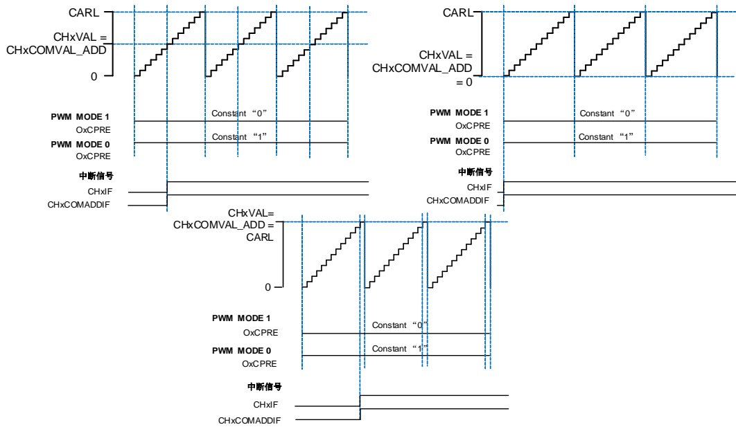
图 24-64. 通道 x 输出 PWM (CHxVAL = CHxCOMVAL_ADD)
