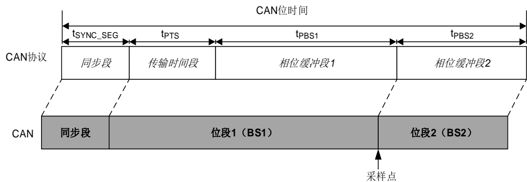
图 42-3. CAN 位时间
