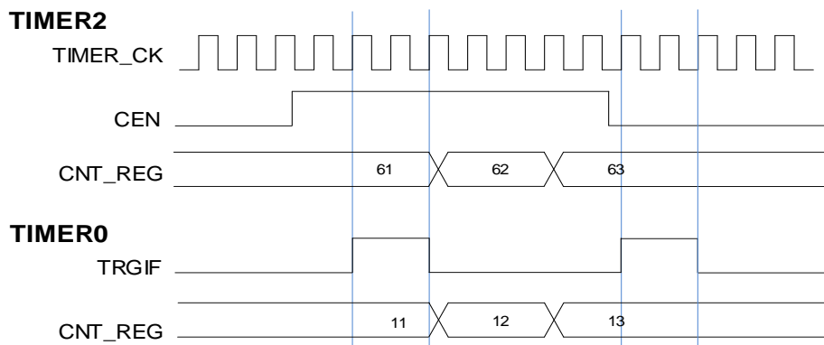
图 24-47. 用定时器 2 的使能来选通定时器 0
