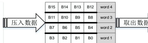
图 16-6. PWIDTH 为‘10’时，数据的打包/解包
