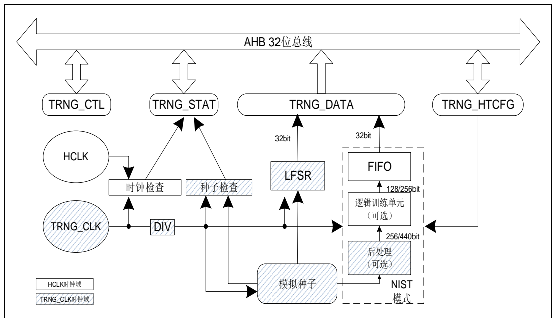
图 12-1. TRNG 模块框图
