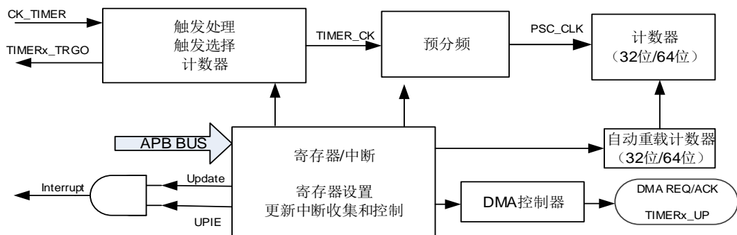
图 24-126. 基本定时器结构框图
