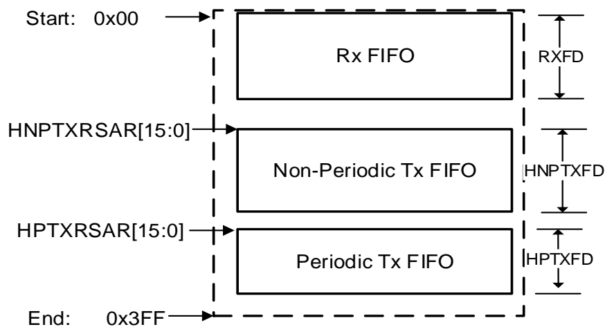
图 49-6. 主机模式 FIFO 空间
