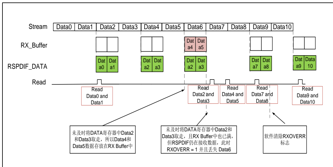
图 33-13. RSPDIF 上溢错误 (RXSTEOMEN = 0 且 RXDF[1:0] = 2'b10)
