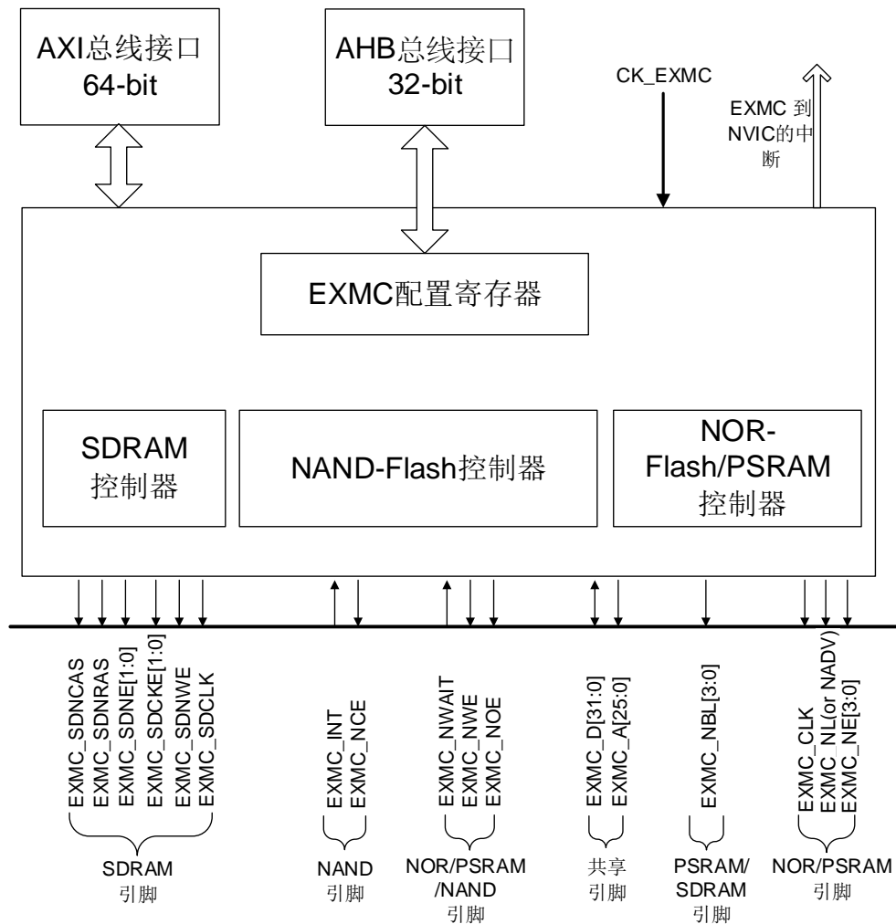
图 38-1. 系统架构
