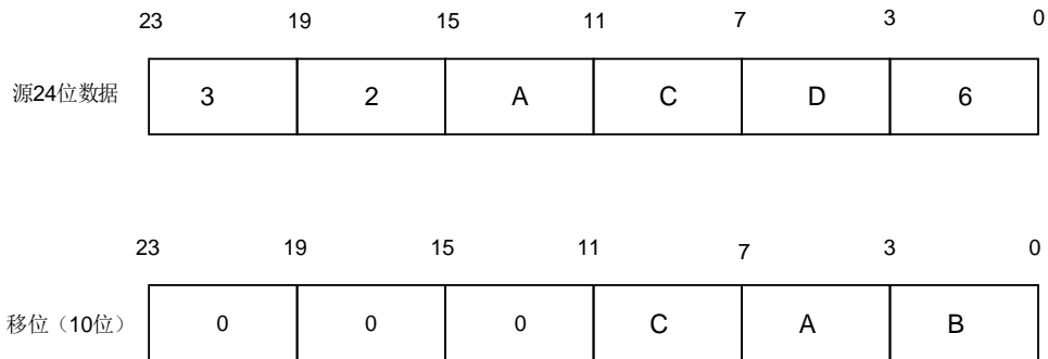
图 20-14. 数值例子 14 位 ADC 过采样右移 10 位
