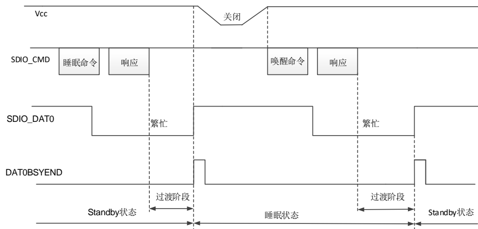
图 36-18. CMD5 时序
