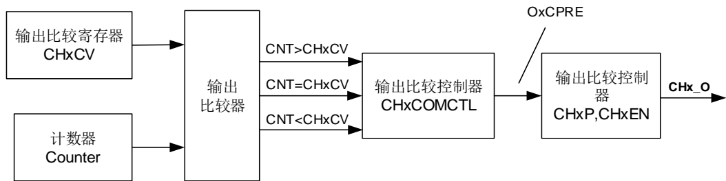
图 24-91. 输出比较逻辑 (x=1)
