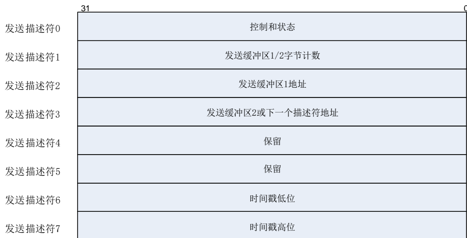
图 43-8. 增强发送描述符
