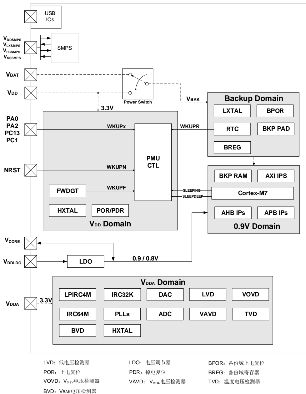
图5-1. 电源域概览
