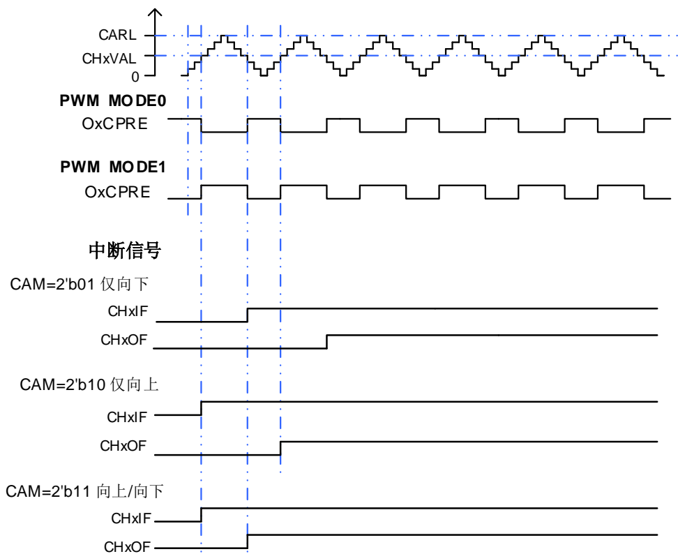
图 24-18. CAPWM 时序图
