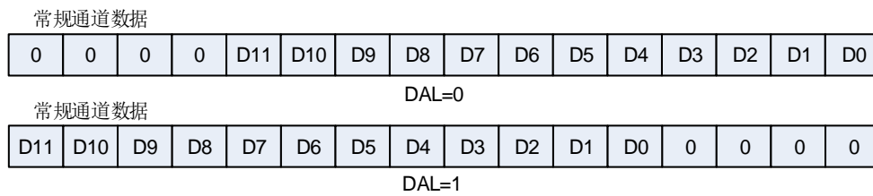
图 20-8. 12 位数据存储模式
