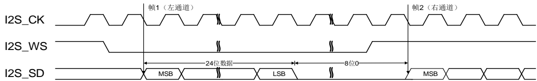
图 27-24. I2S 飞利浦标准时序图 (DTLEN = 01, CHLEN = 1, CKPL = 0)
