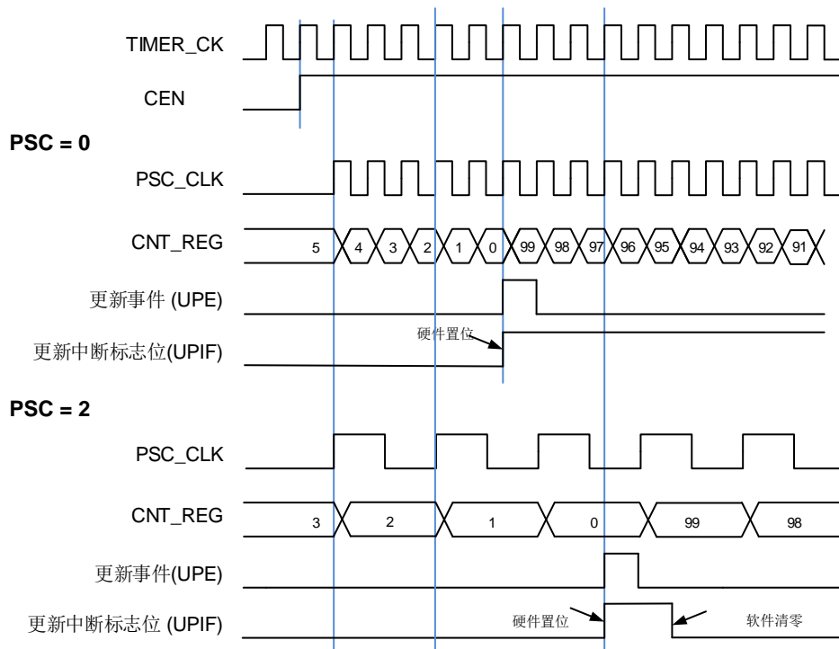
图 24-55. 向下计数时序图, PSC=0/2
