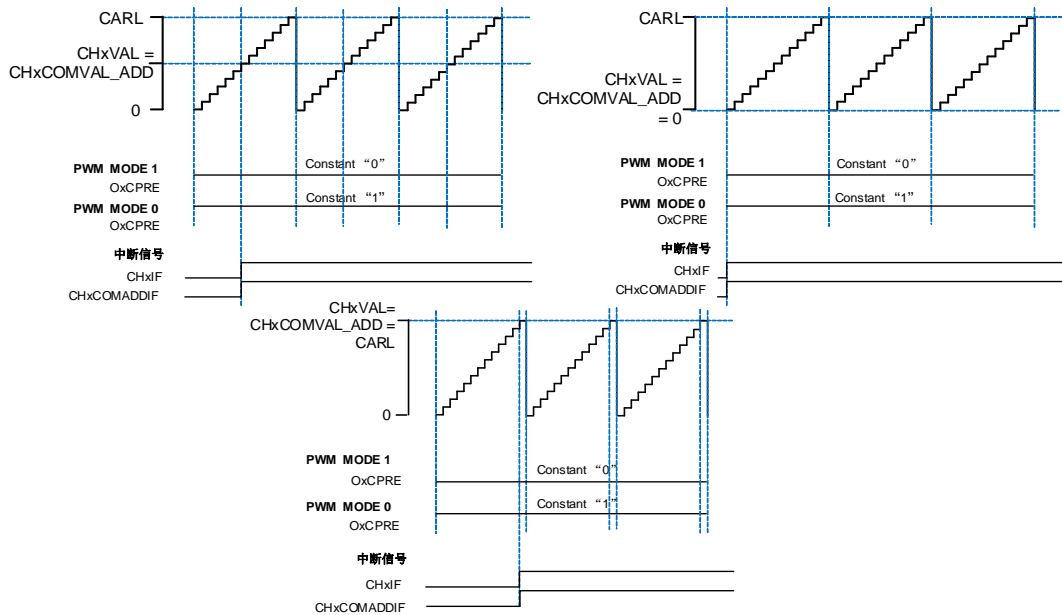
图 24-20. 通道 x 输出 PWM (CHxVAL = CHxCOMVAL_ADD)
