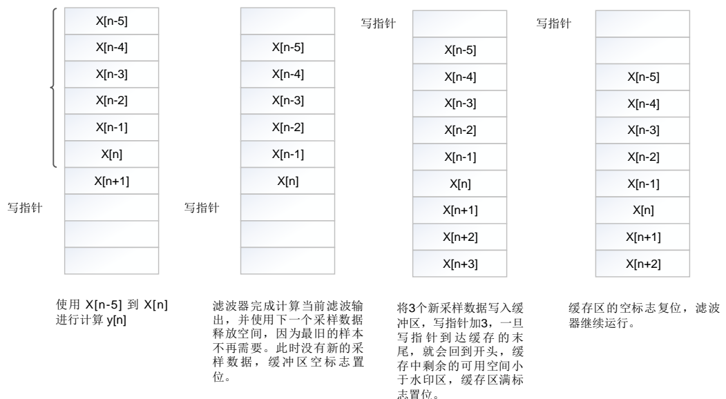
图 47-4. 循环输入缓冲区区域
