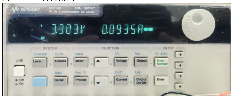
图 5-3. Rx 功耗测试
